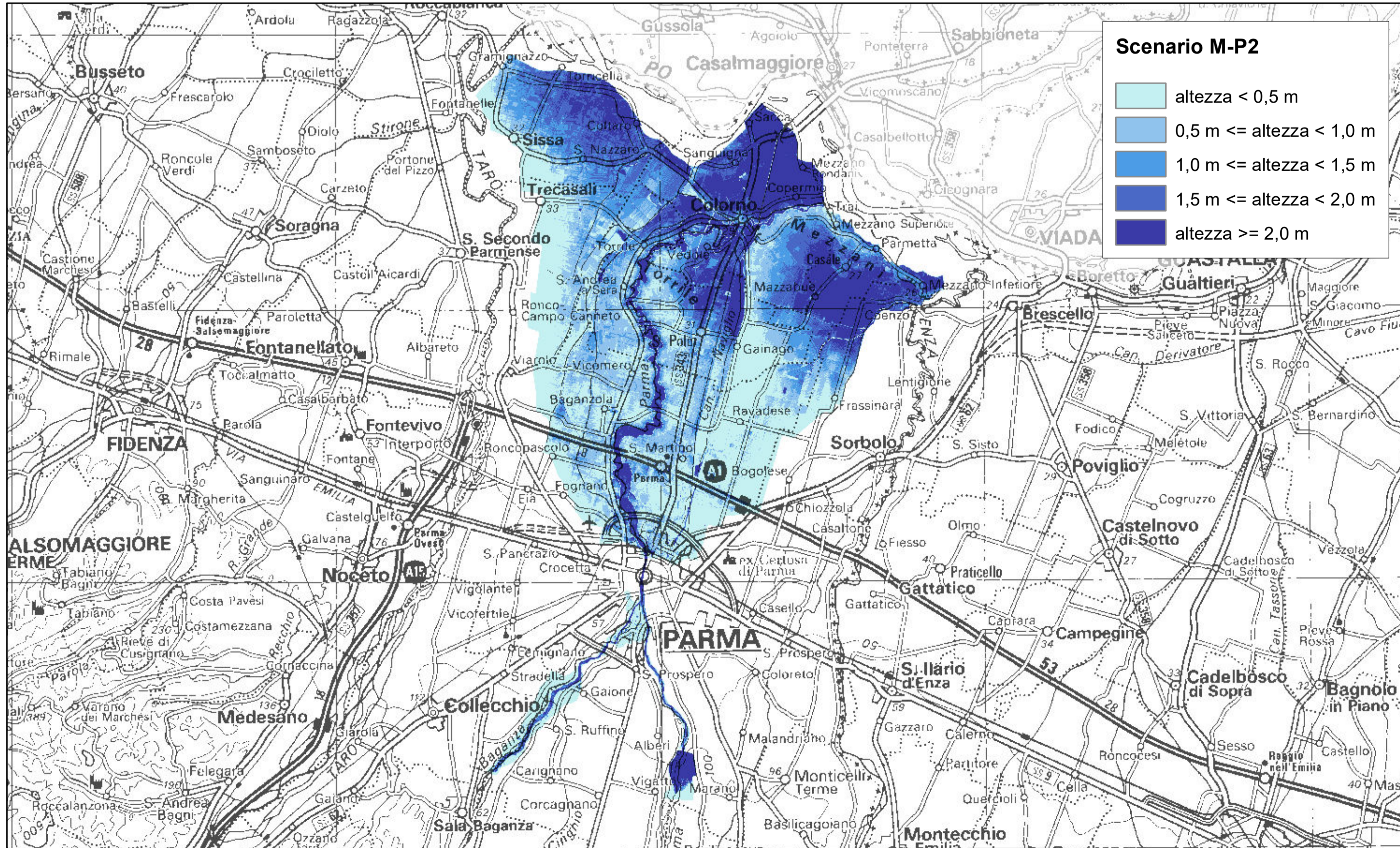
Scenario di media probabilità (M-P2)
