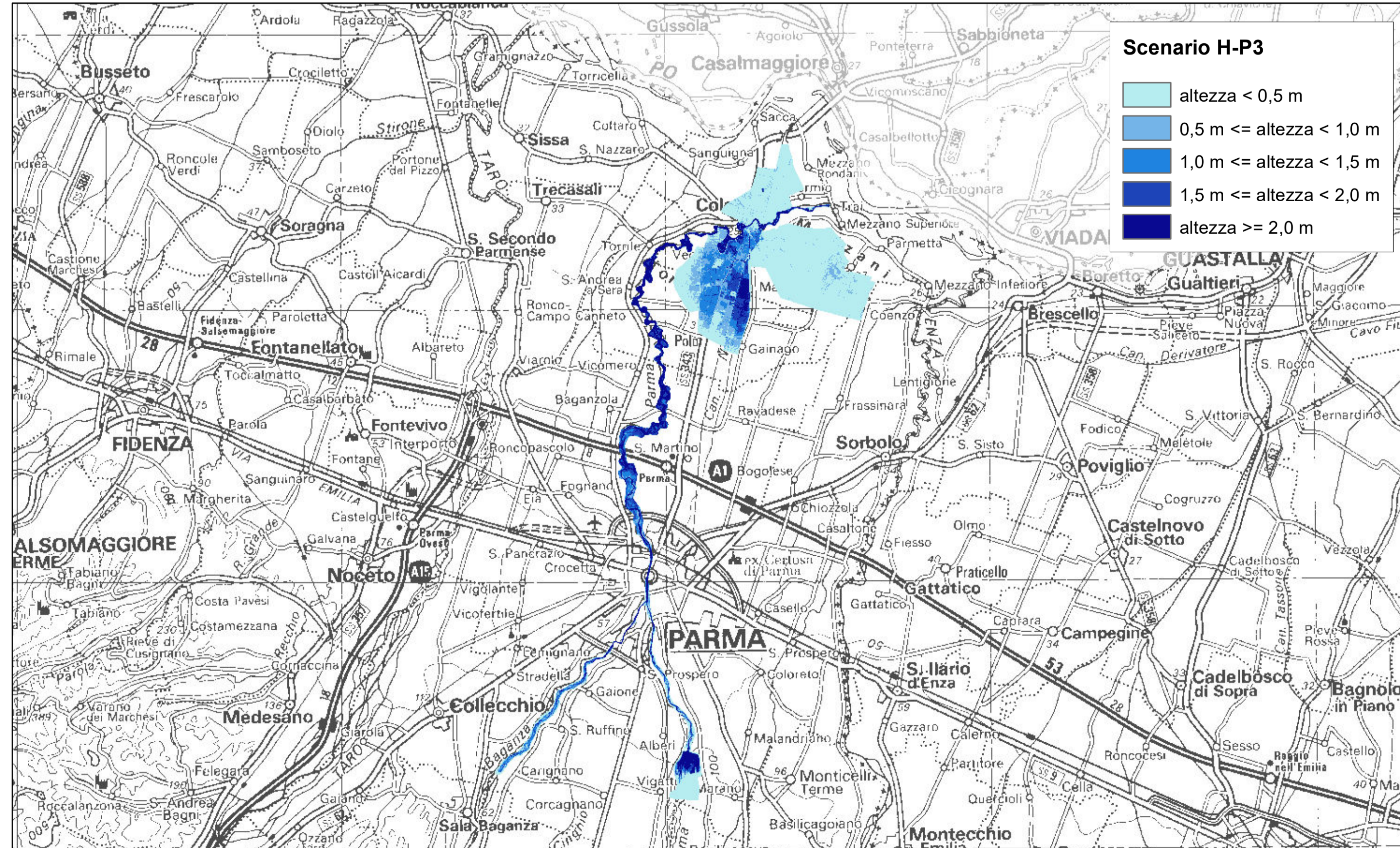
Scenario di elevata probabilità (H-P3)
