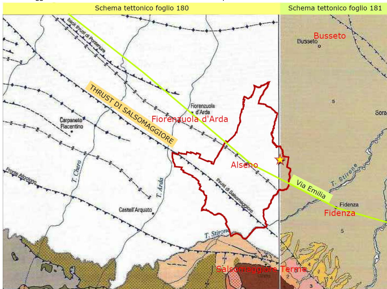
Figura 2.3. Estratto dagli schemi tettonici dei Fogli 180 e 181 della Carta Geologica d'Italia alla scala 1:50.000. In evidenza il thrust di Salsomaggiore che attraversa il territorio comunale [con la stella gialla è indicato l'ultimo terremoto registrato ricadente all'interno del territorio comunale - 30/07/2007].
