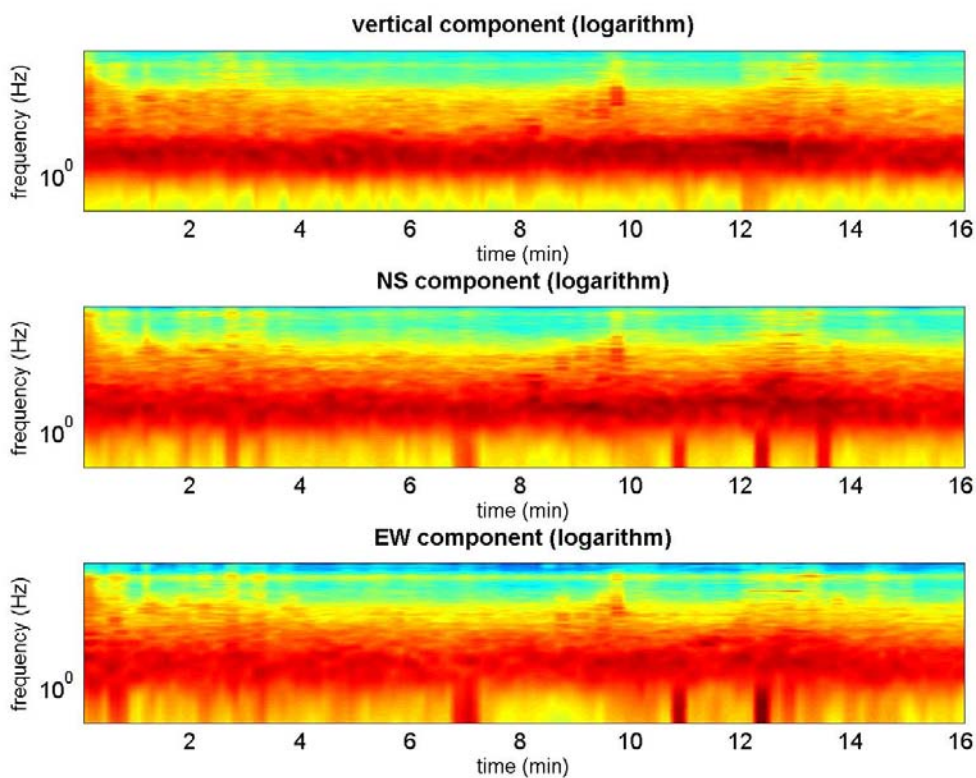
Figura 7. Persistenza delle misure HVSR lungo le singole componenti.
