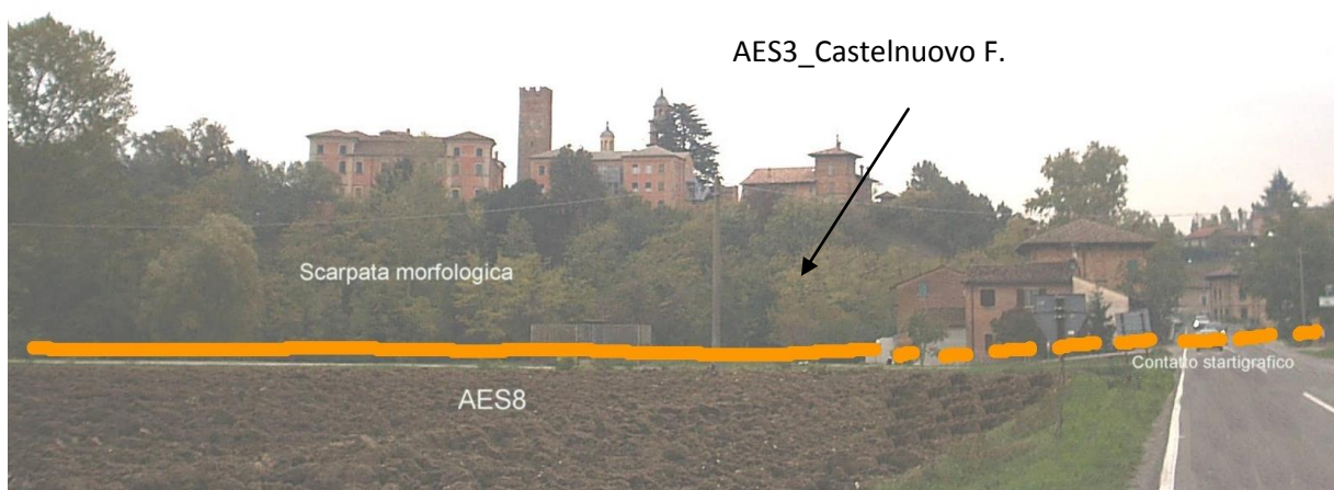
Figura 3.3 Vista del terrazzo “rissiano” (AES3) di Castelnuovo F.
