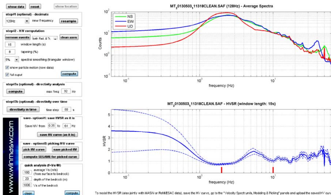
Figura 9. Spettri d'ampiezza medi delle 3 componenti (NS, EW e verticale) e valori di HVSR.
