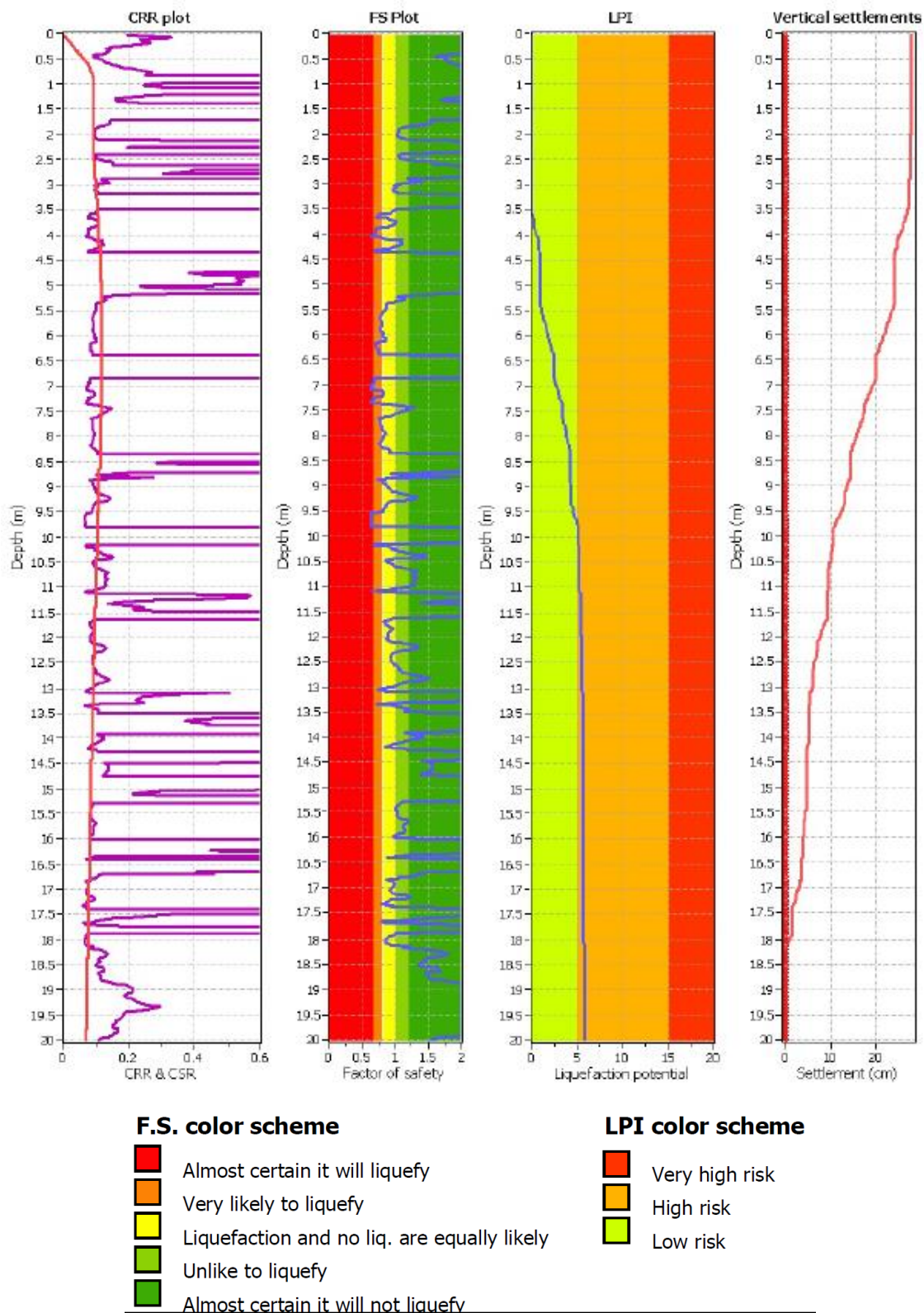
Fig. 35 – Grafici di CSR-CRR, dei fattori di sicurezza FS, dell'indice di liquefazione (LPI), e del cedimento valutati per la prova CPTU_1
