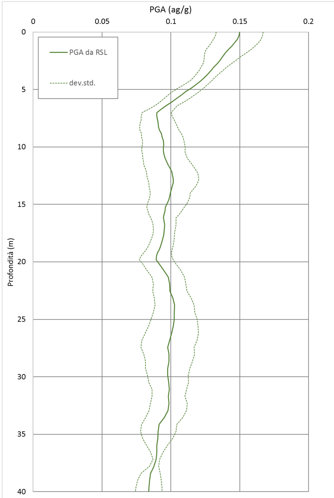
Fig. 30 - Variazione dell'accelerazione con la profondità
