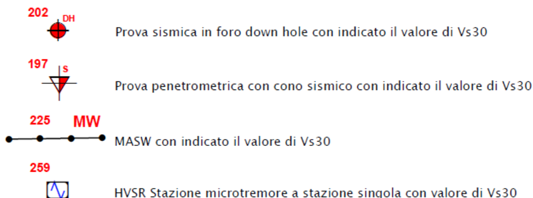
Fig. 16 - Legenda della Carta delle velocità delle onde di taglio S ( V_s )
