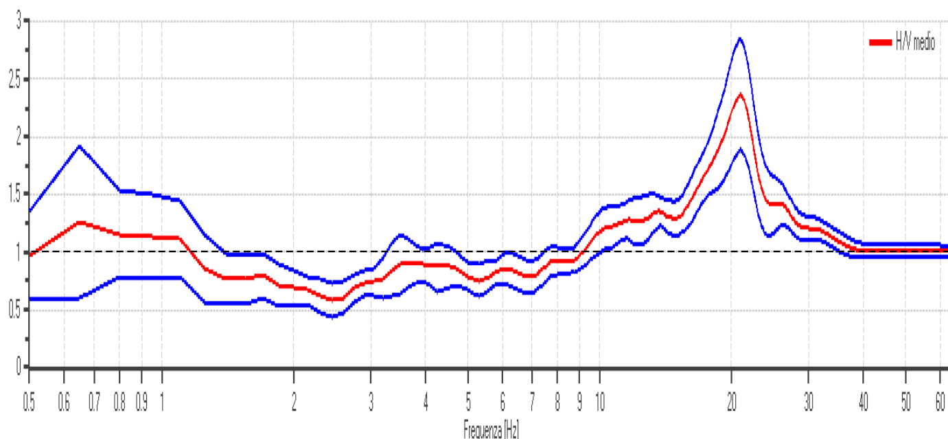
Fig. 9 - Esempio di curva H/V naturale con curva H/V sintetica
