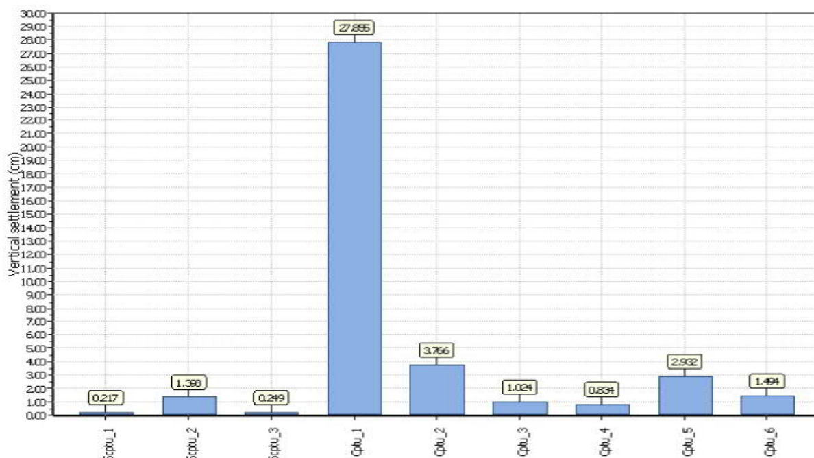
Fig. 37 - Riepilogo dei cedimenti attesi per tutte le prove
