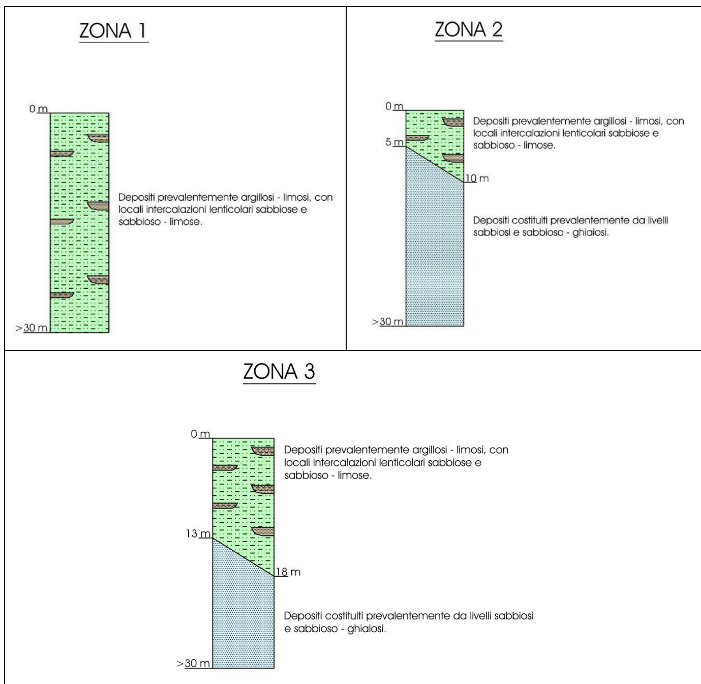
Fig. 15 - Colonne litostratigrafiche sintetiche, rappresentative della microzone
