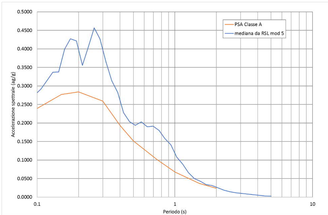
Fig. 28 - Confronto tra gli spettri elastici in accelerazione
