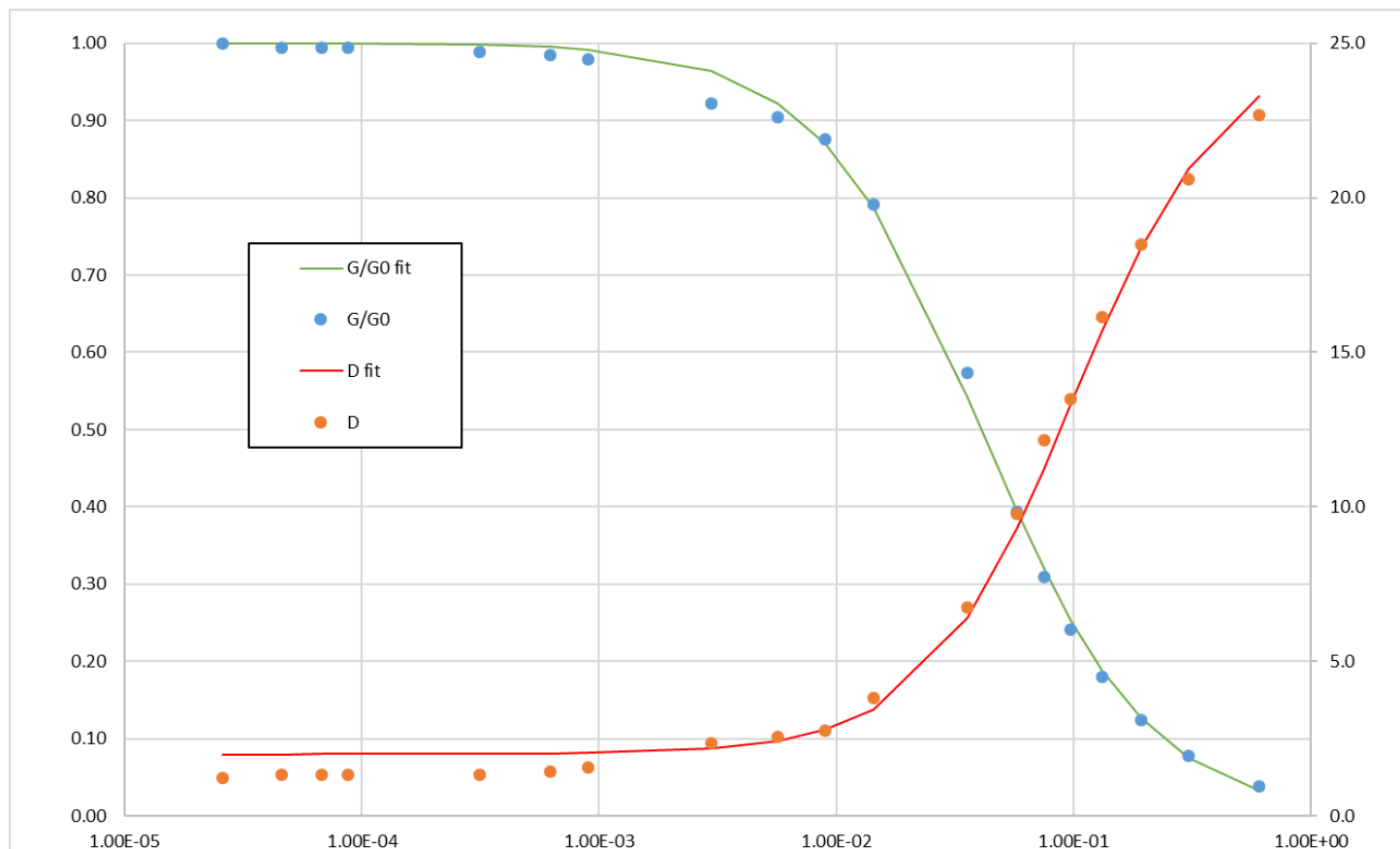
Fig. 23 - Grafico dei dati sperimentali e delle curve di interpolazione per il campione S1SH2
