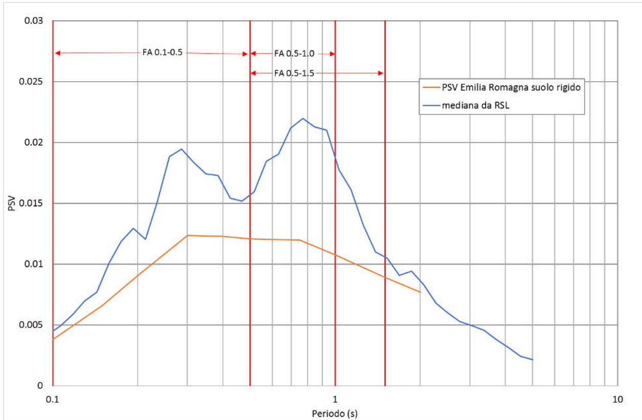
Fig. 29 - Confronto tra gli spettri elastici in velocità
