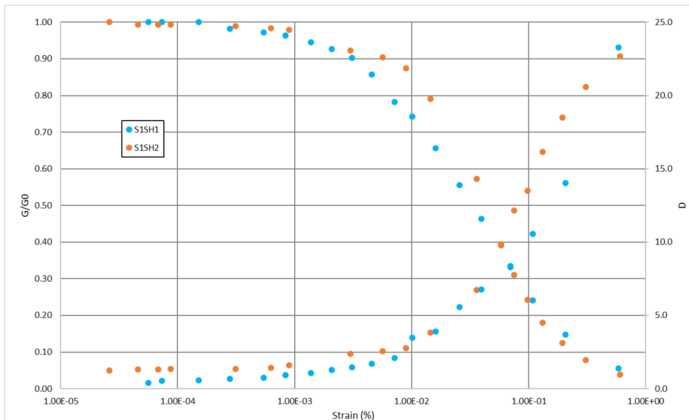
Fig. 22 - Dati sperimentali delle prove RC
