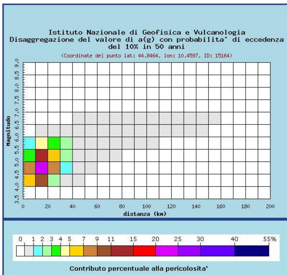
Fig. 32 - Disaggregazione magnitudo-distanza per il nodo 15164
