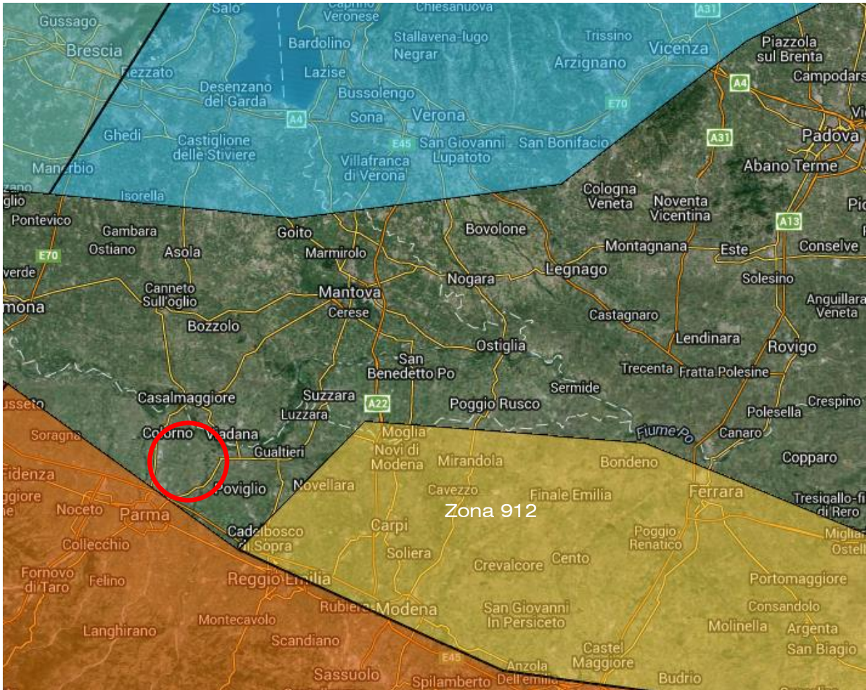
Fig. 34 - Classificazione ZS9
