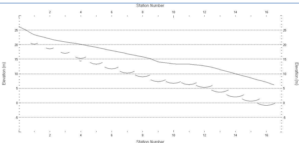
Sovrapposizione del metodo classico al profilo tomografico
