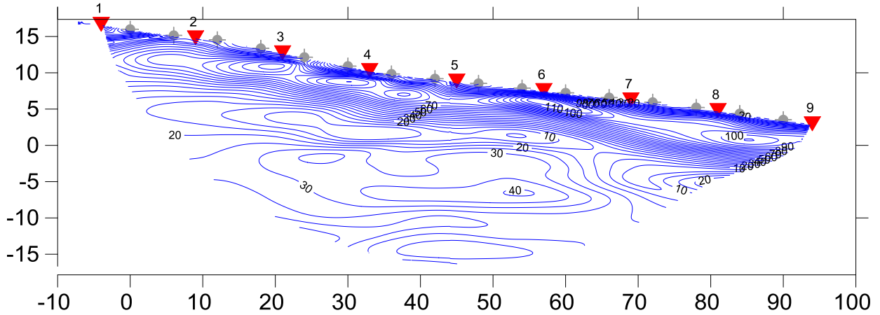
Mappa di gradiente di velocità
