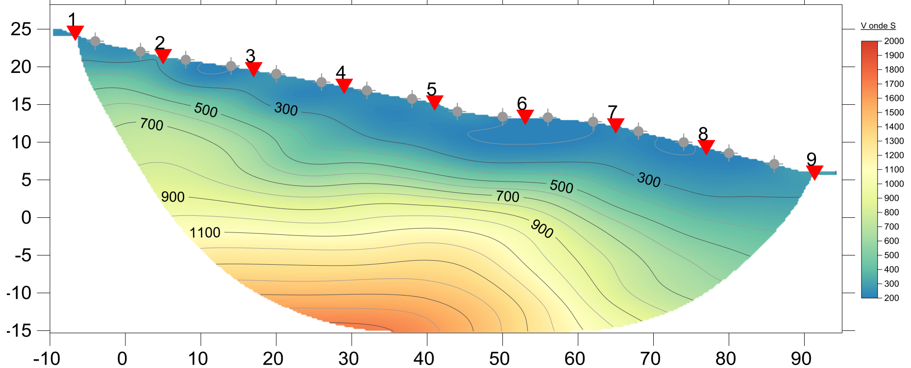
Tomografia sismica in onde S
