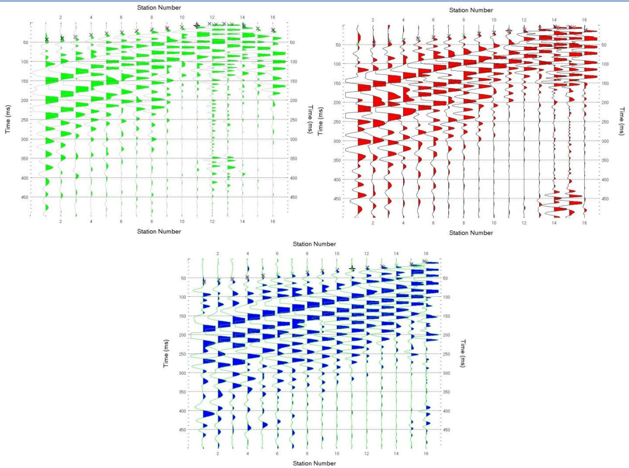
Dromocrone sperimentali (solo tratteggio) e sintetiche (contrassegnate con la x)
