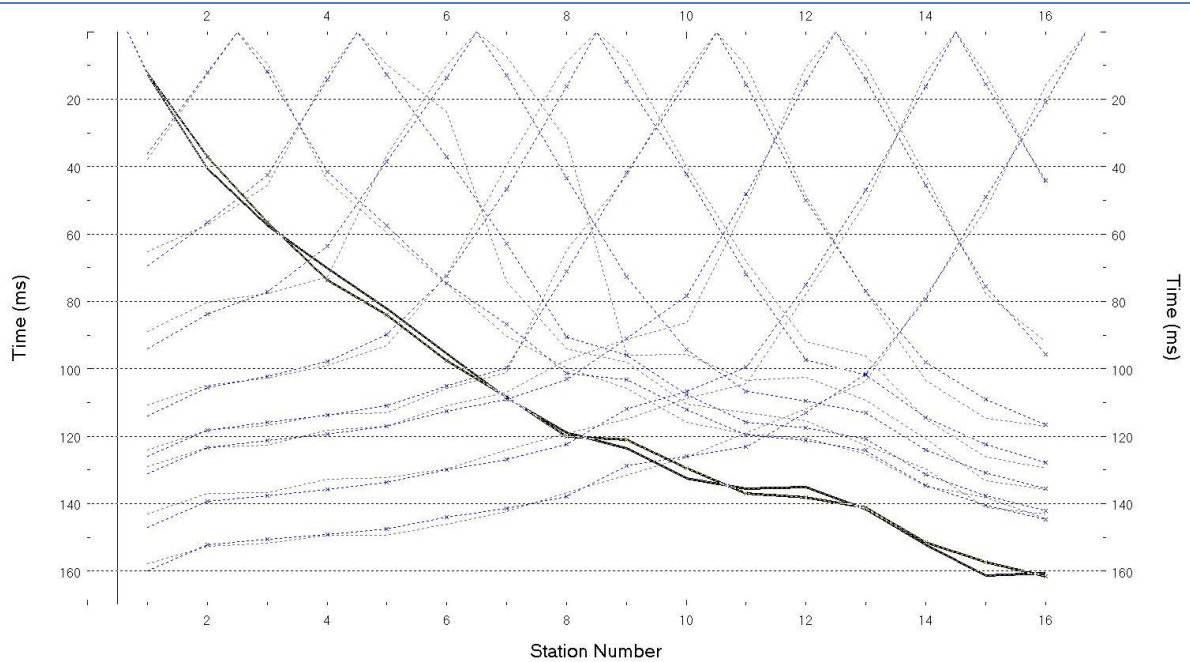
Dromocrone sperimentali e sintetiche (contrassegnate con la x)
