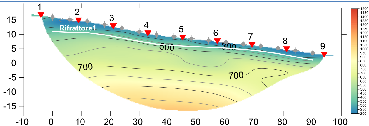
Sovrapposizione del metodo classico al profilo tomografico
