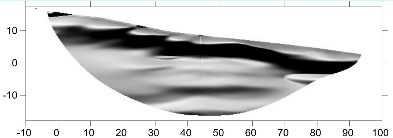
Shade map del gradiente di velocità
