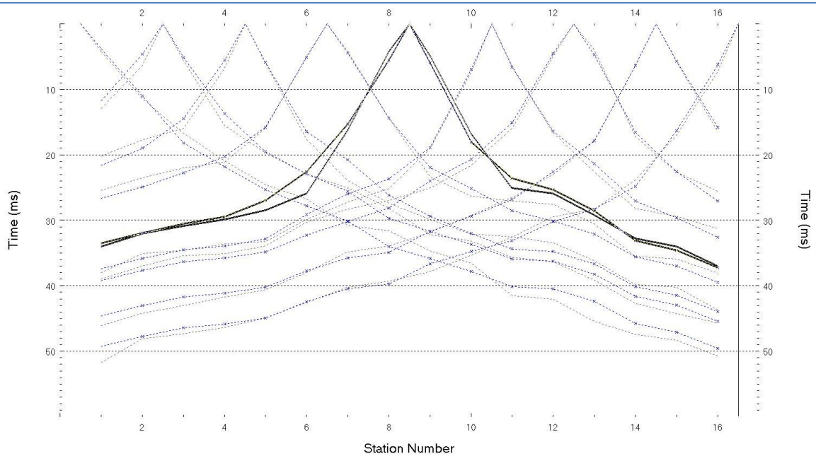
Dromocrone sperimentali (solo tratteggio) e sintetiche (contrassegnate con la x)
