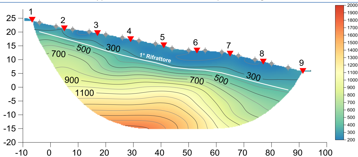
Sovrapposizione del metodo classico al profilo tomografico
