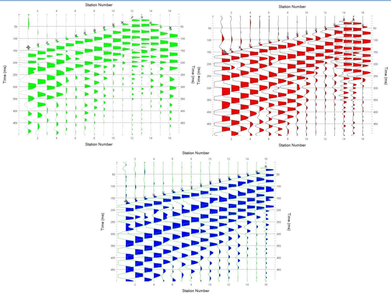
Dromocrone sperimentali e sintetiche (contrassegnate con la x)
