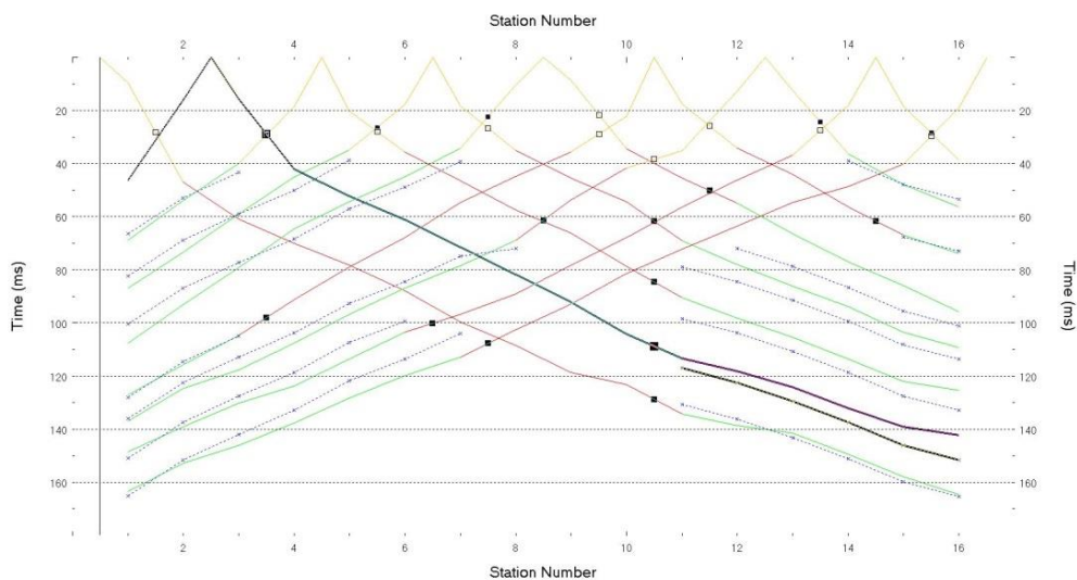
Profilo in elevazione ottenuto mediante metodo Plus-minus
