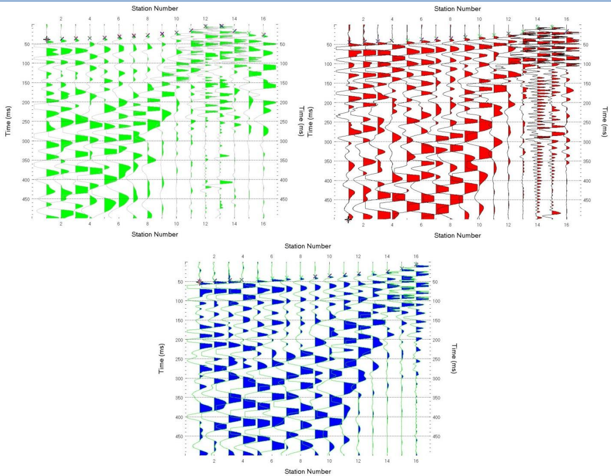
Dromocrone sperimentali (solo tratteggio) e sintetiche (contrassegnate con la x)
