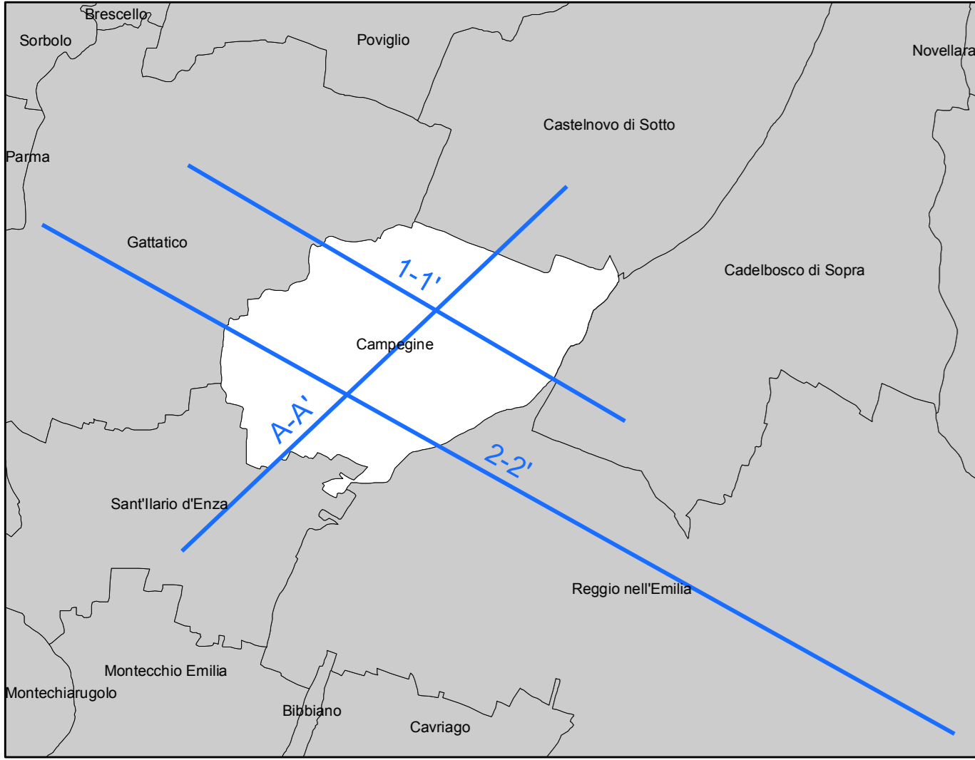
1 - 1' Traccia della sezione geologica 1 - 1' (Scala distanze 1:25.000 - Scala altezze 1:1.000)
