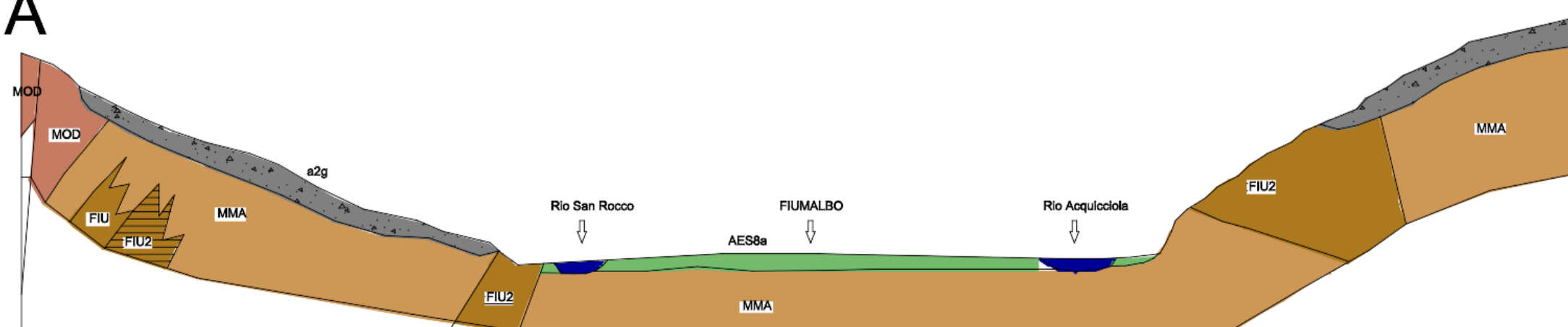
Sezione 2 - scala 1:2.000
