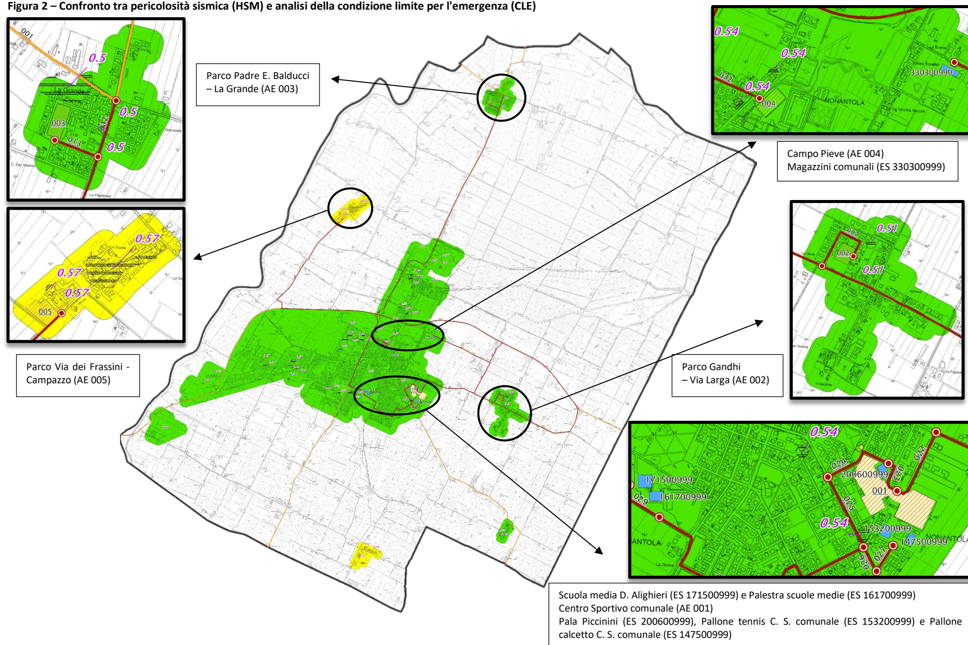
Figura 2 – Confronto tra pericolosità sismica (HSM) e analisi della condizione limite per l'emergenza (CLE)
