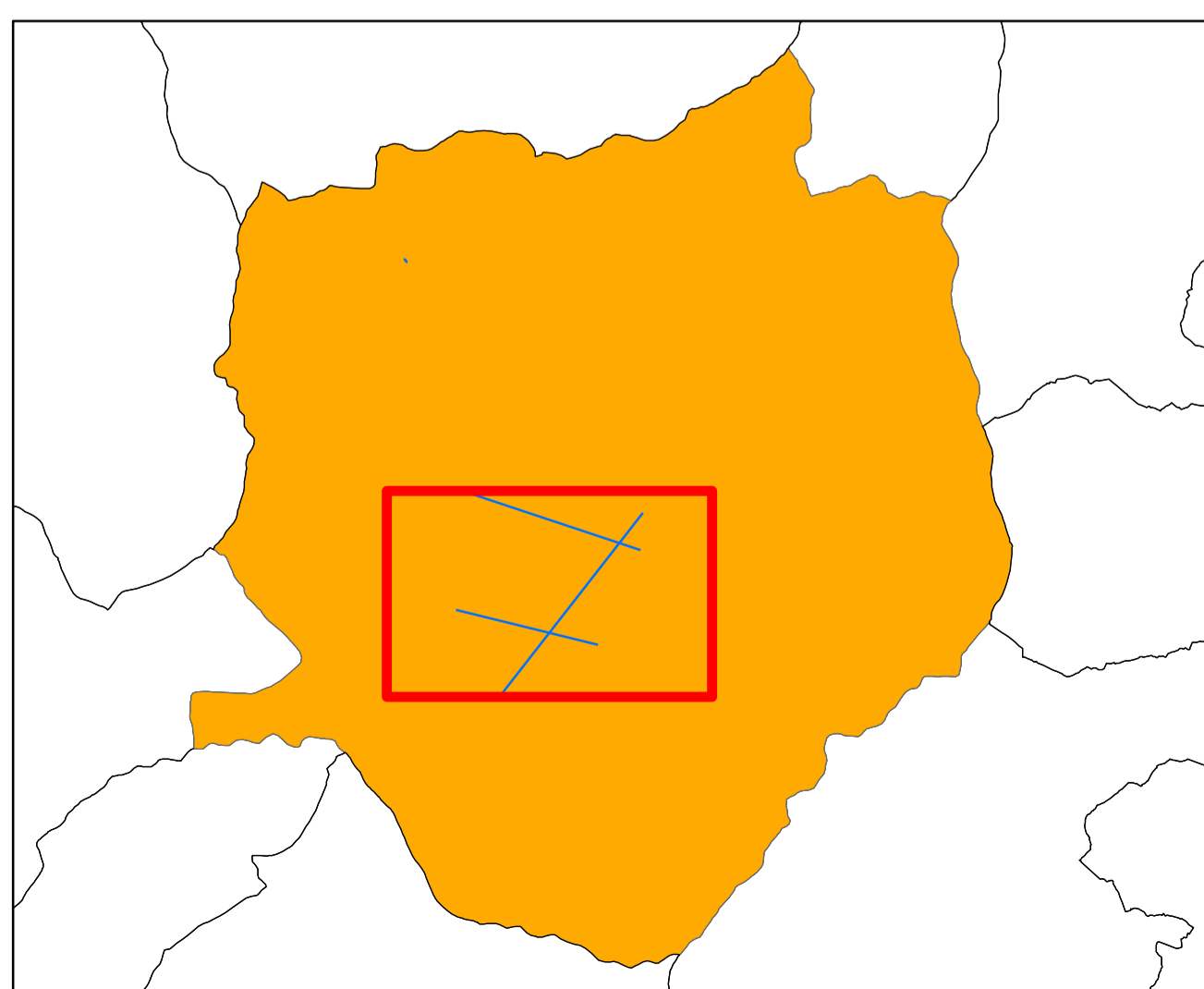
SEZIONE QUERCIAGIROSSA W-E
