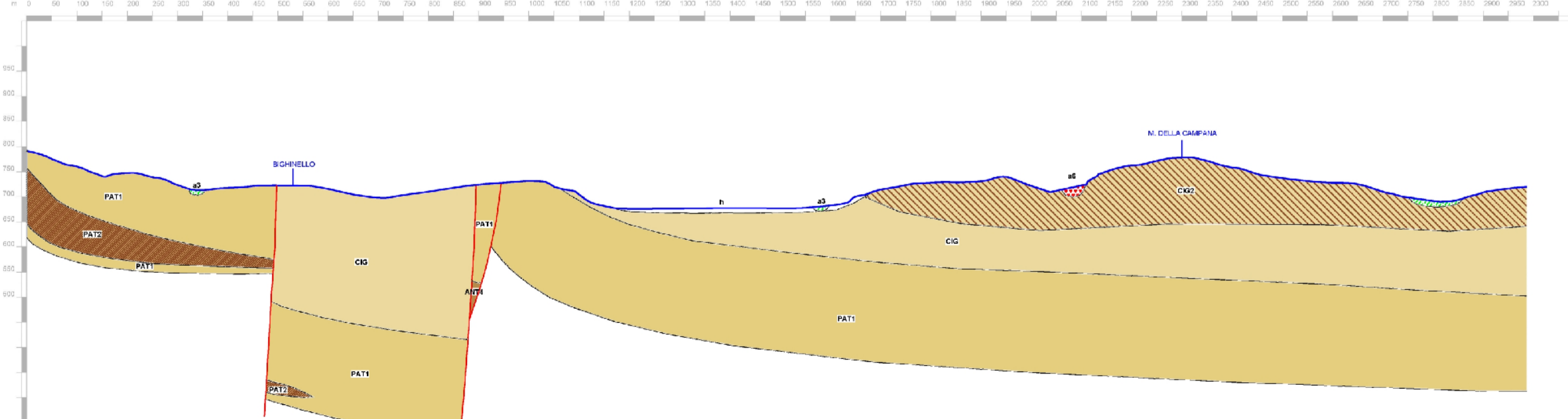
SEZIONE PAVULLO NEL FRIGNANO W-E
