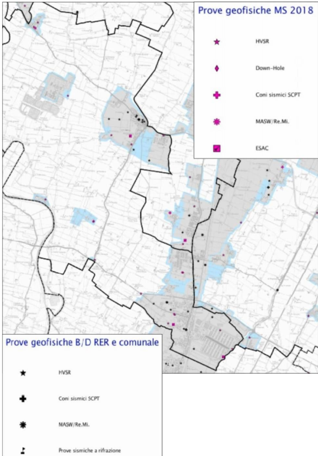
Figura 4.2- Localizzazione delle indagini geofisiche (di repertorio e di nuova esecuzione) disponibili per lo studio di microzonazione sismica
