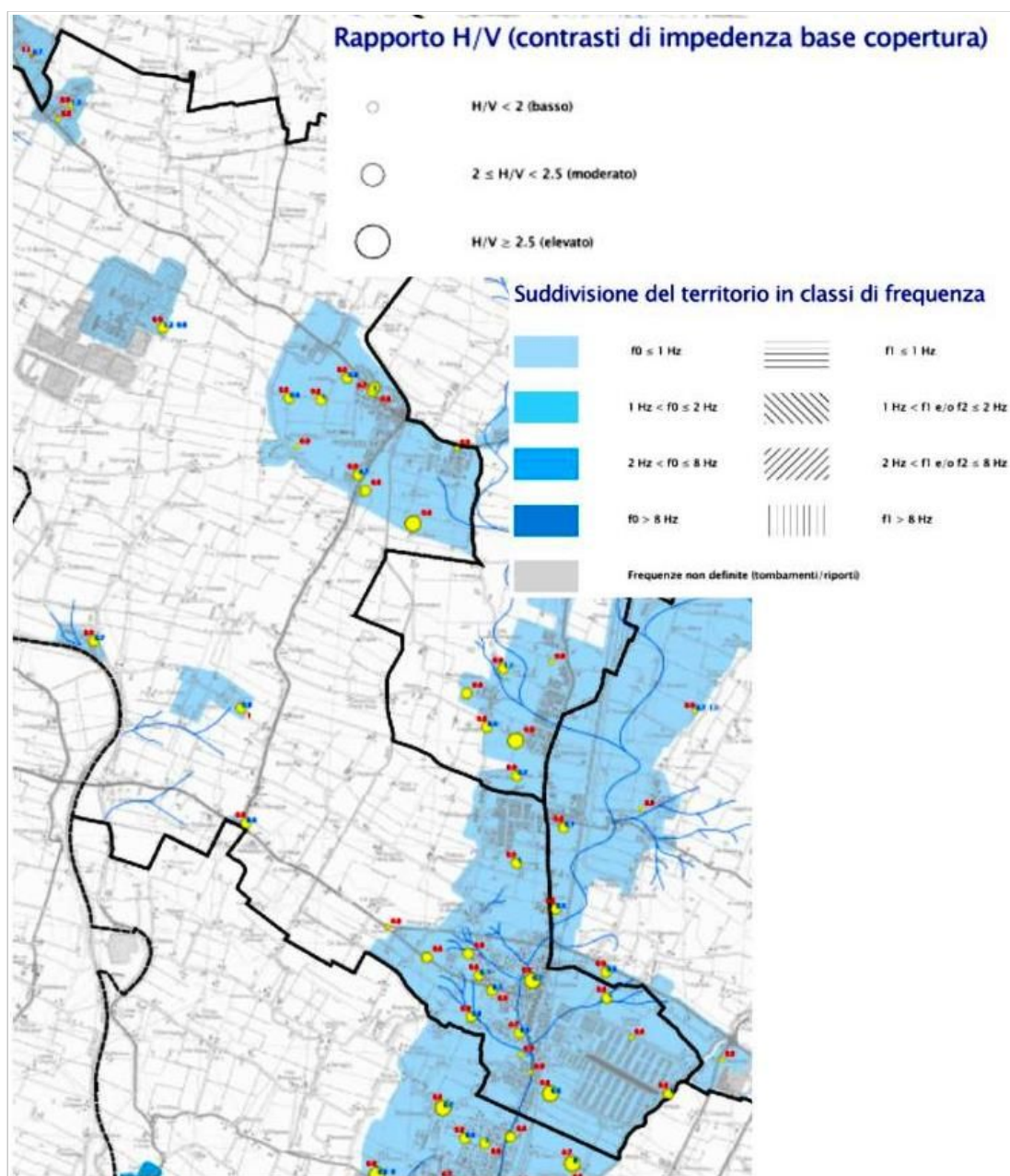
Figura 5.10 – Suddivisione del territorio urbano/urbanizzabile di Argelato in classi di frequenza naturale dei terreni. I colori rappresentano classi differenti. L'ampiezza dei cerchi classifica le massime amplificazioni spettrali ricavate dalle registrazioni HVSR
