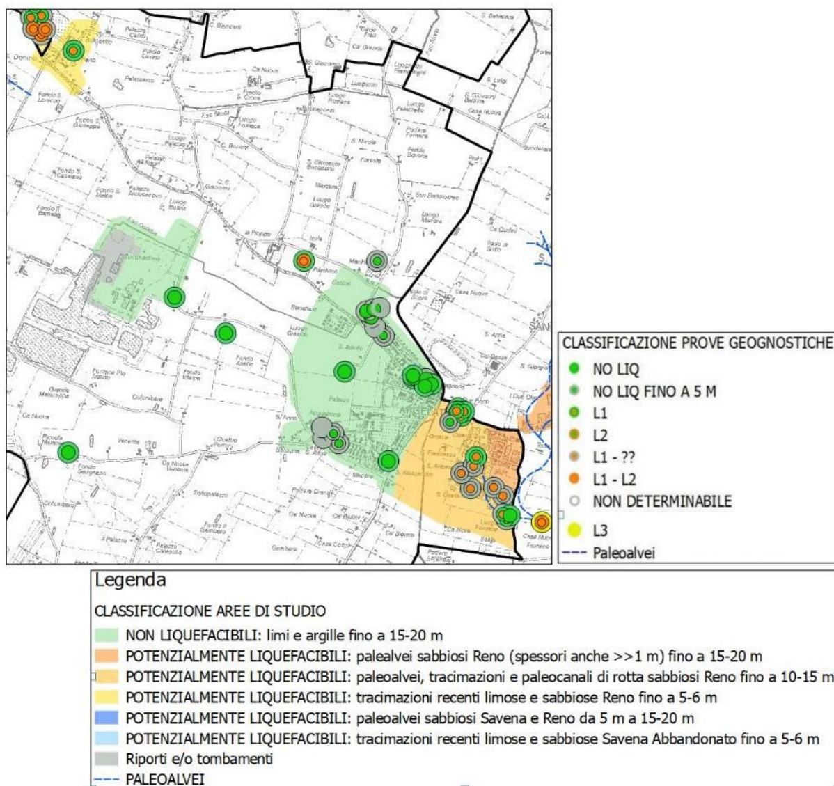
Figura 6.4 - Classificazione dei punti di controllo geognostici finalizzata alla ricostruzione delle zone di potenziale liquefacibilità in base alla presenza di strati granulari in falda. Territorio comunale nord
