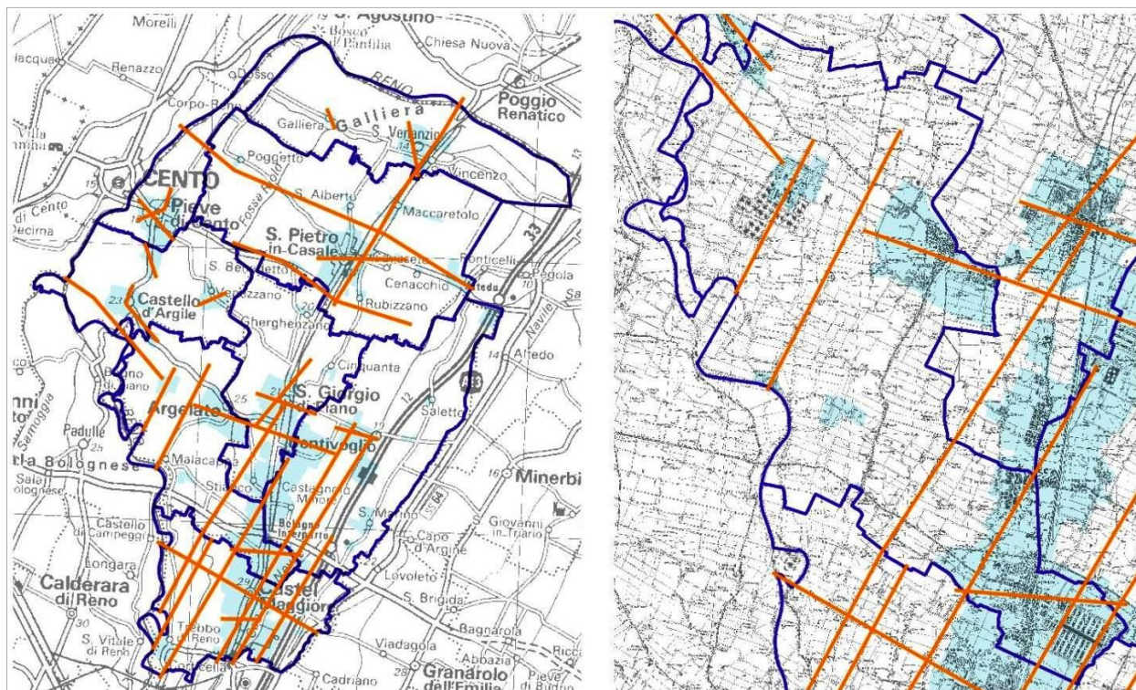
Figura 5.3 - Sezioni litotecniche di riferimento per lo studio di MS (Unione Reno Galliera e dettaglio di Argelato)
