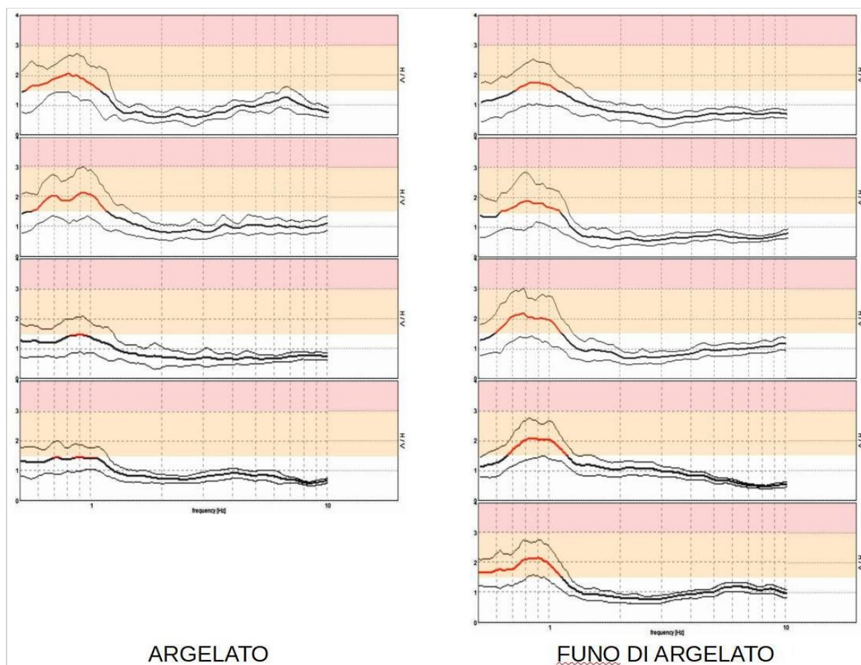
Figura 5.11 – Confronto tra spettri H/V ricavati da registrazioni HVSR nel Comune di Argelato
