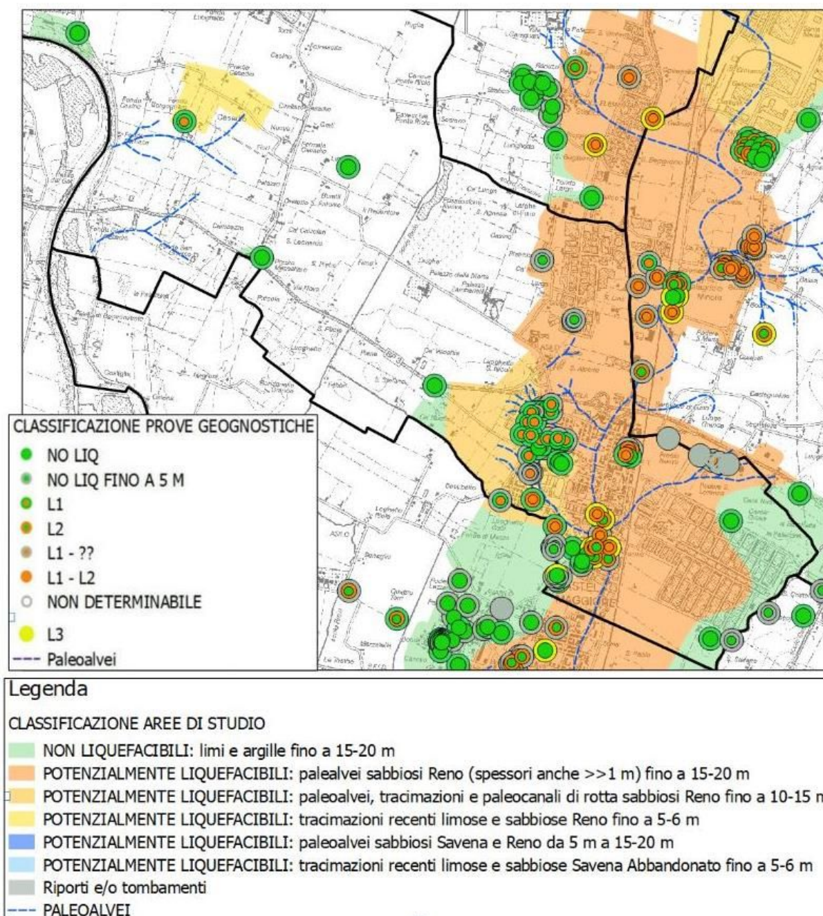
Figura 6.3 - Classificazione dei punti di controllo geognostici finalizzata alla ricostruzione delle zone di potenziale liquefaccibilità in base alla presenza di strati granulari in falda. Territorio comunale sud
