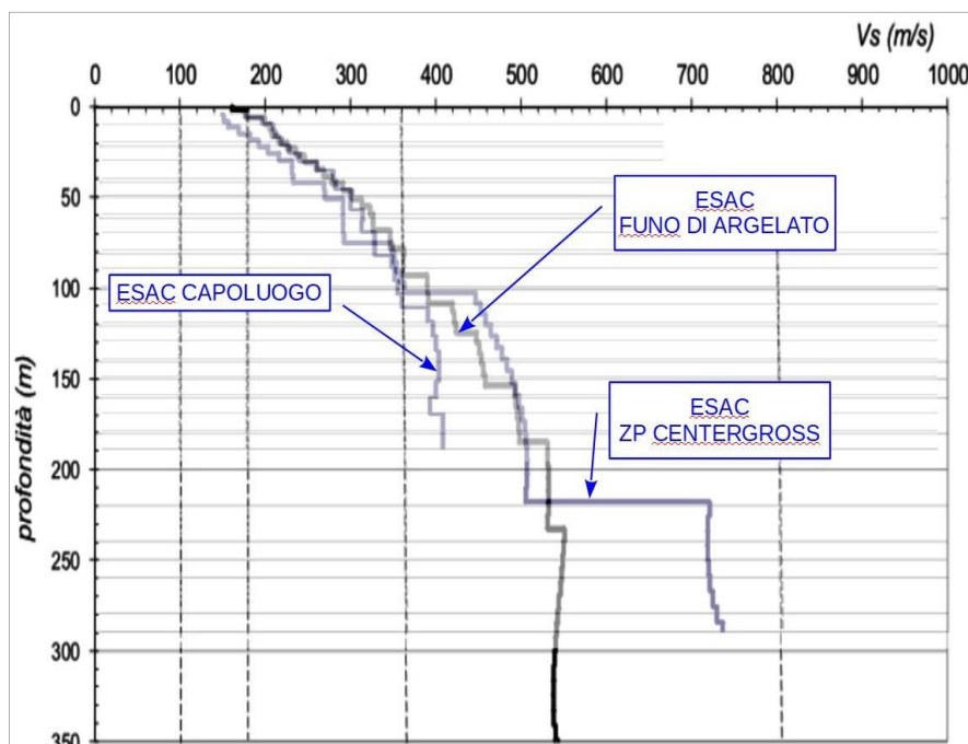
Figura 5.8- Sismostratigrafie ricavate dagli stendimenti ESAC eseguiti nel territorio di Argelato (Capoluogo; Funo e ZP Centergross)
