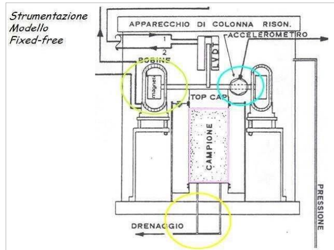
Figura 4.3- Schema della colonna risonante di tipo "Fixed - free" (fonte: sito ISMGEO)
