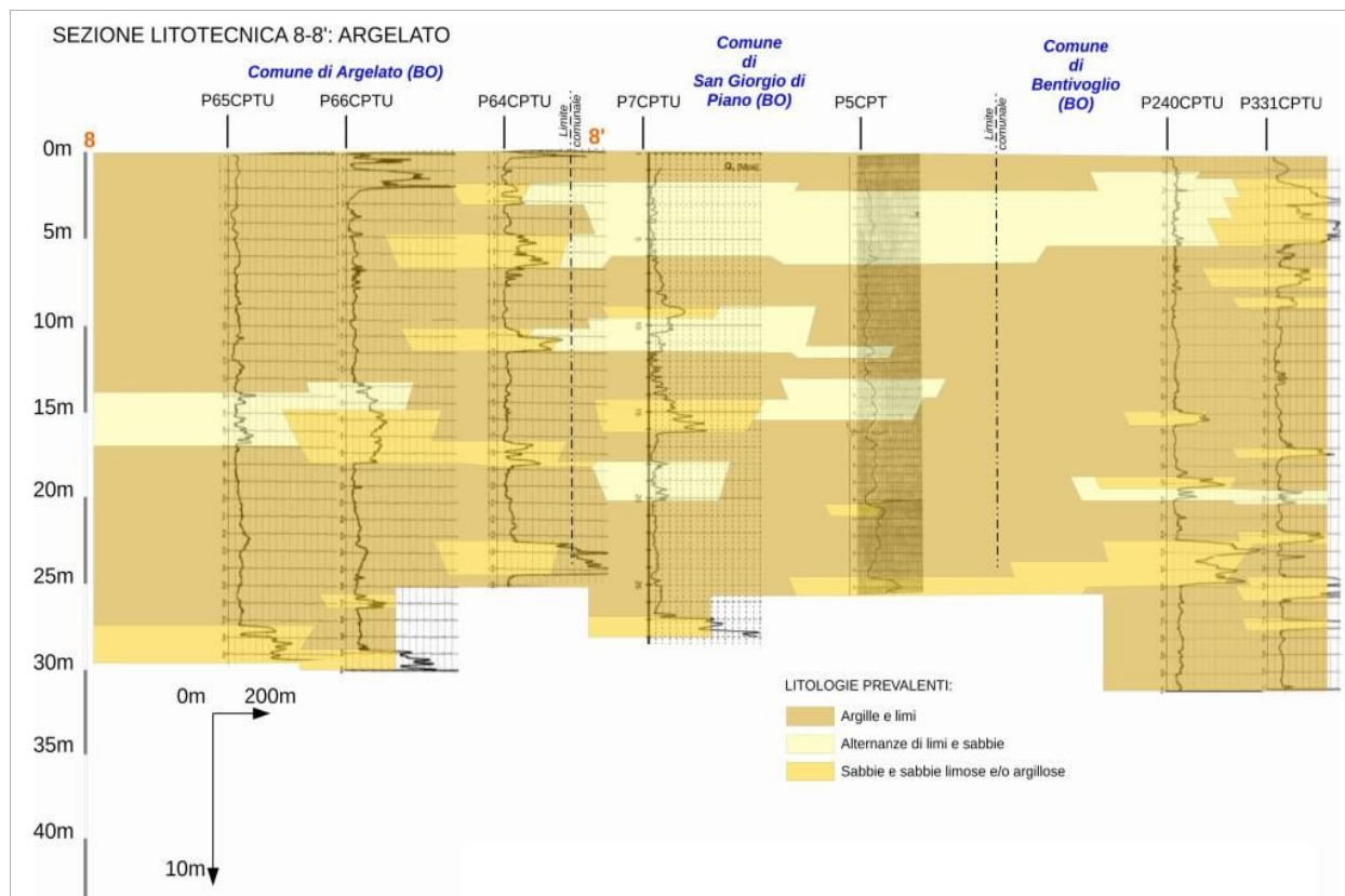
Figura 5.5- Sezione litotecnica 8-8' (Capoluogo) elaborata per questo studio
