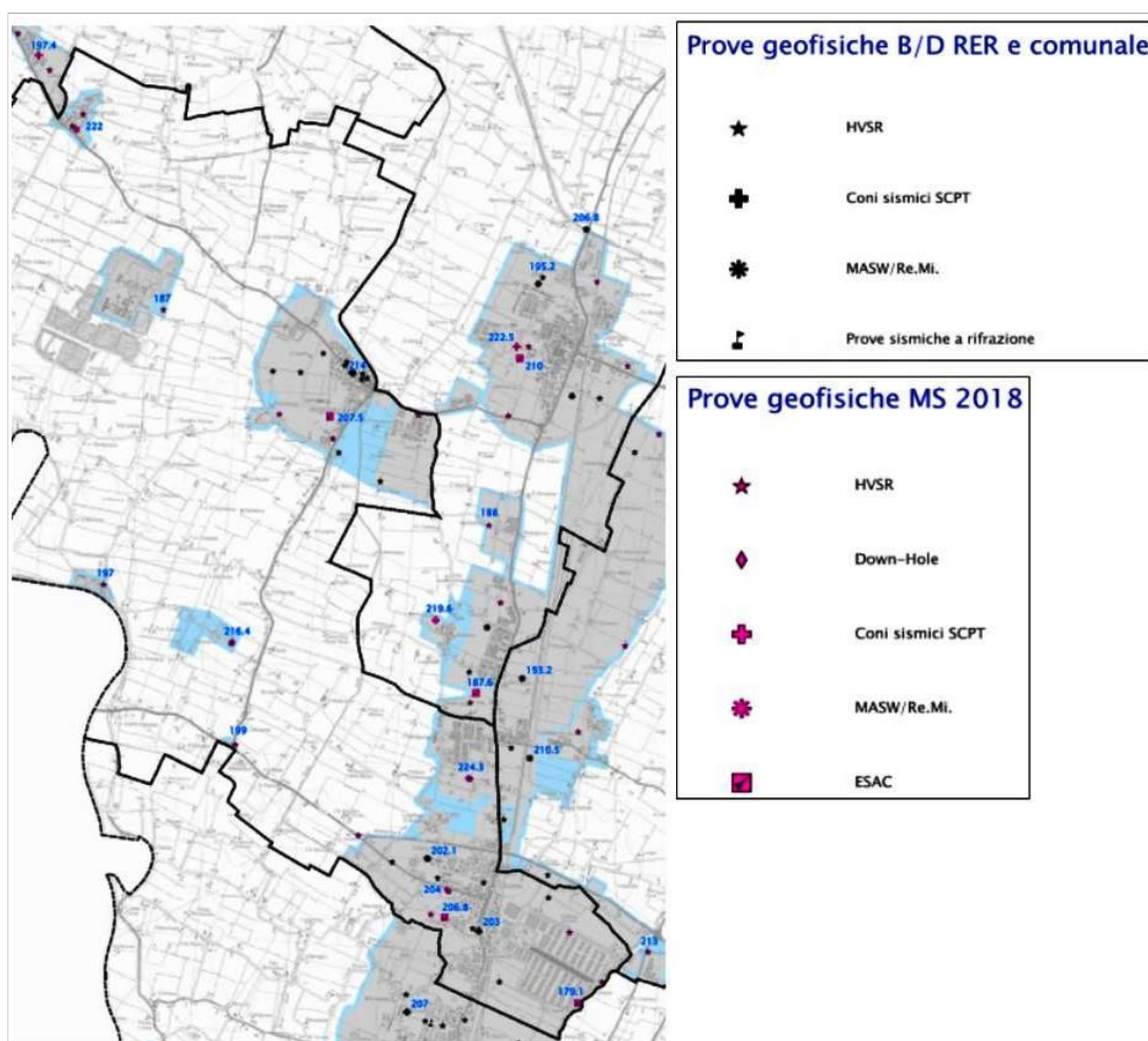
Figura 5.9 - Indagini geofisiche disponibili nel territorio di Argelato con calcolo della Vs30. È indicata anche la tipologia di prova
