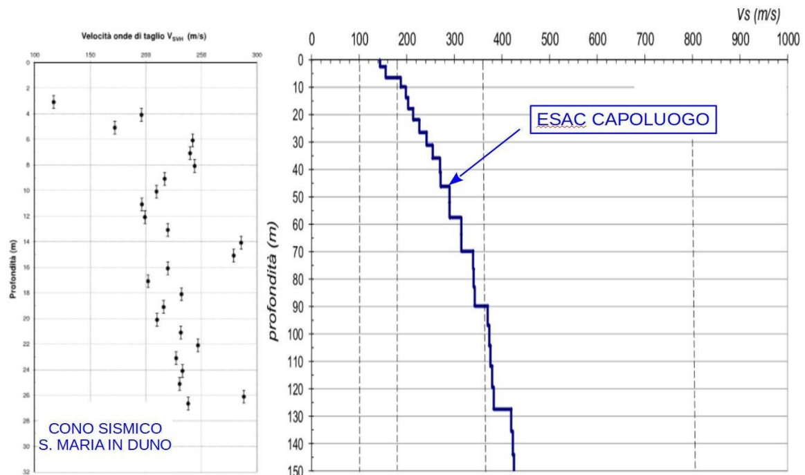
Figura 5.8- Sismostratigrafie ricavate dal "Cono Sismico" eseguito nella frazione S. Maria in Duno e dallo stendimento ESAC eseguito nel Capoluogo
