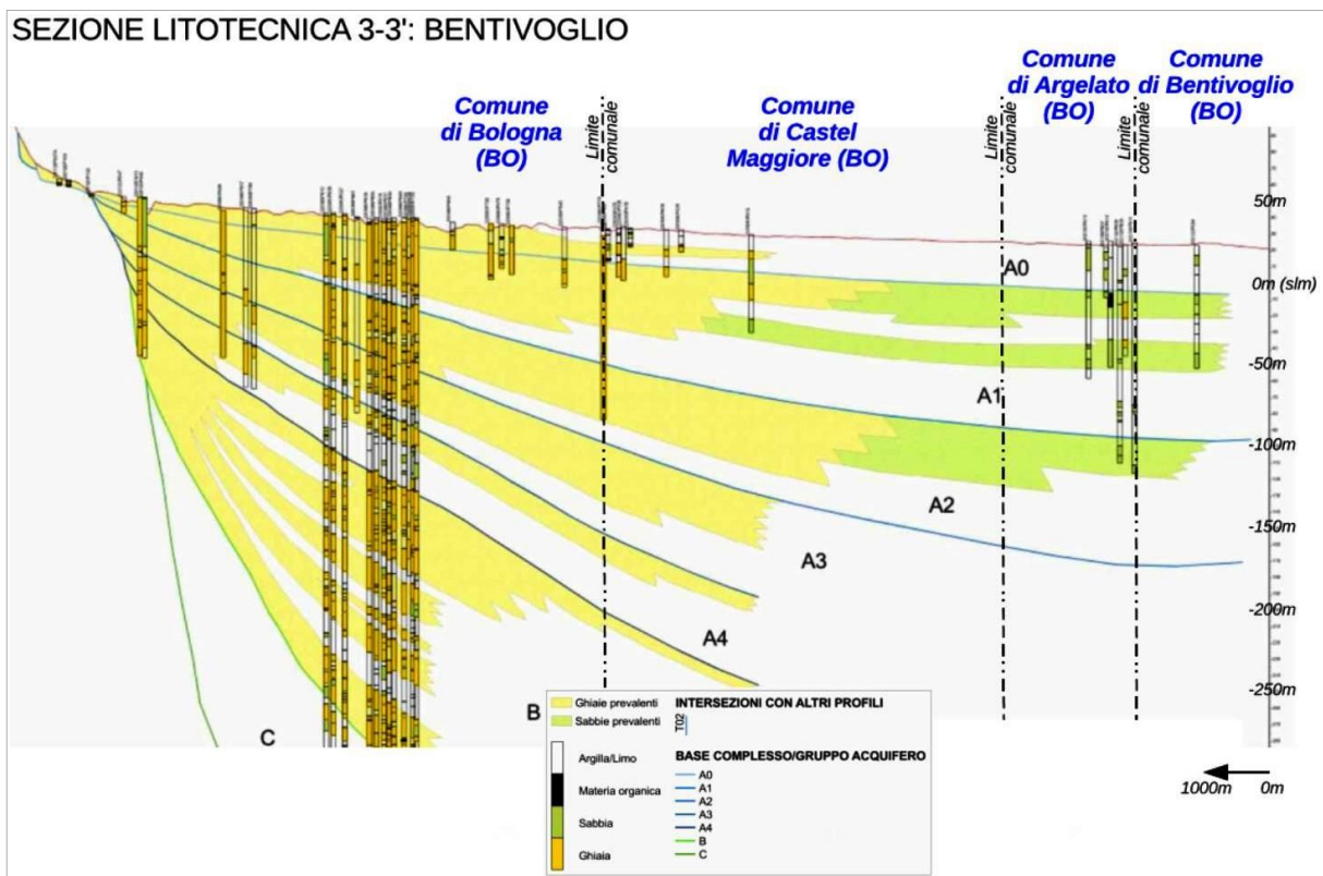
Figura 5.4 – Sezione litotecnica RER (rinominata 3-3' per questo studio)
