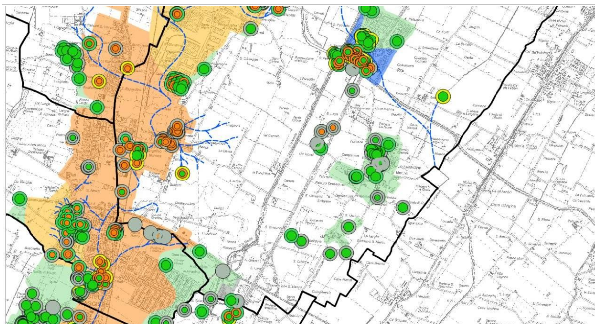
Figura 6.4 - Classificazione dei punti di controllo geognostici finalizzata alla ricostruzione delle zone di potenziale liquefabilità in base alla presenza di strati granulari in falda (territorio SUD)
