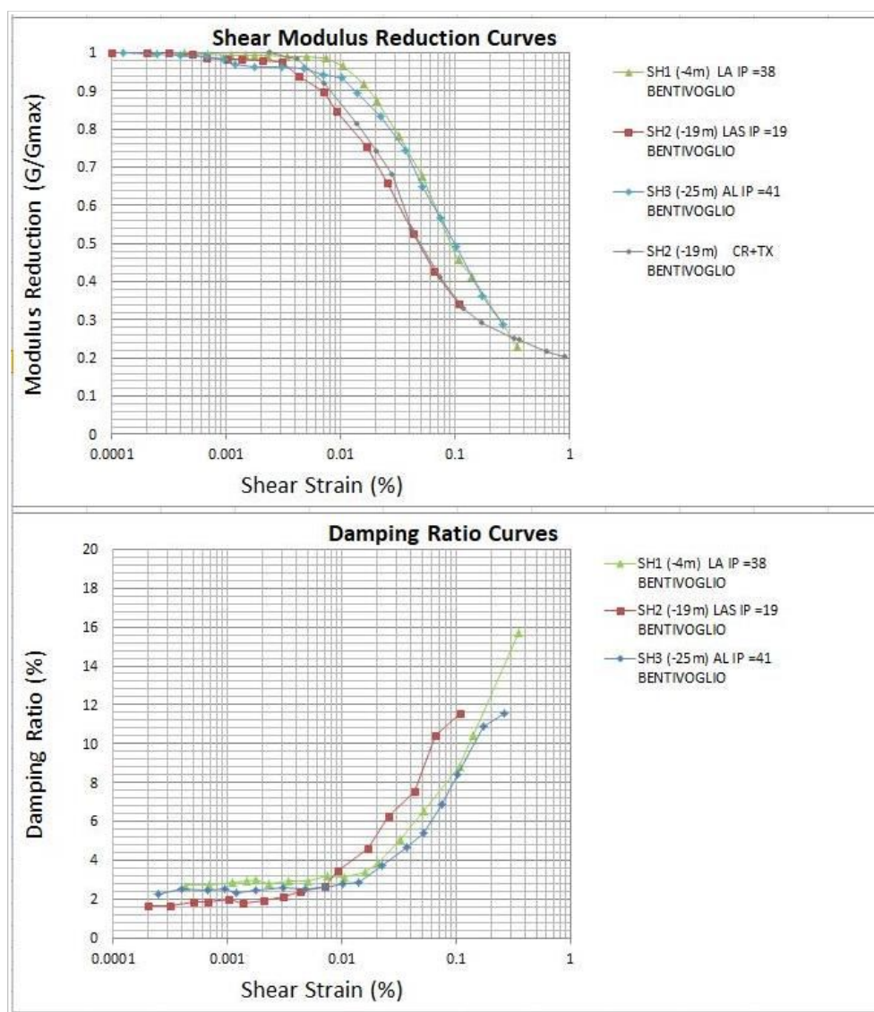
Figura 5.2 - Curve di decadimento dei sedimenti fini di Bentivoglio (sondaggio eseguito nel Capoluogo)
