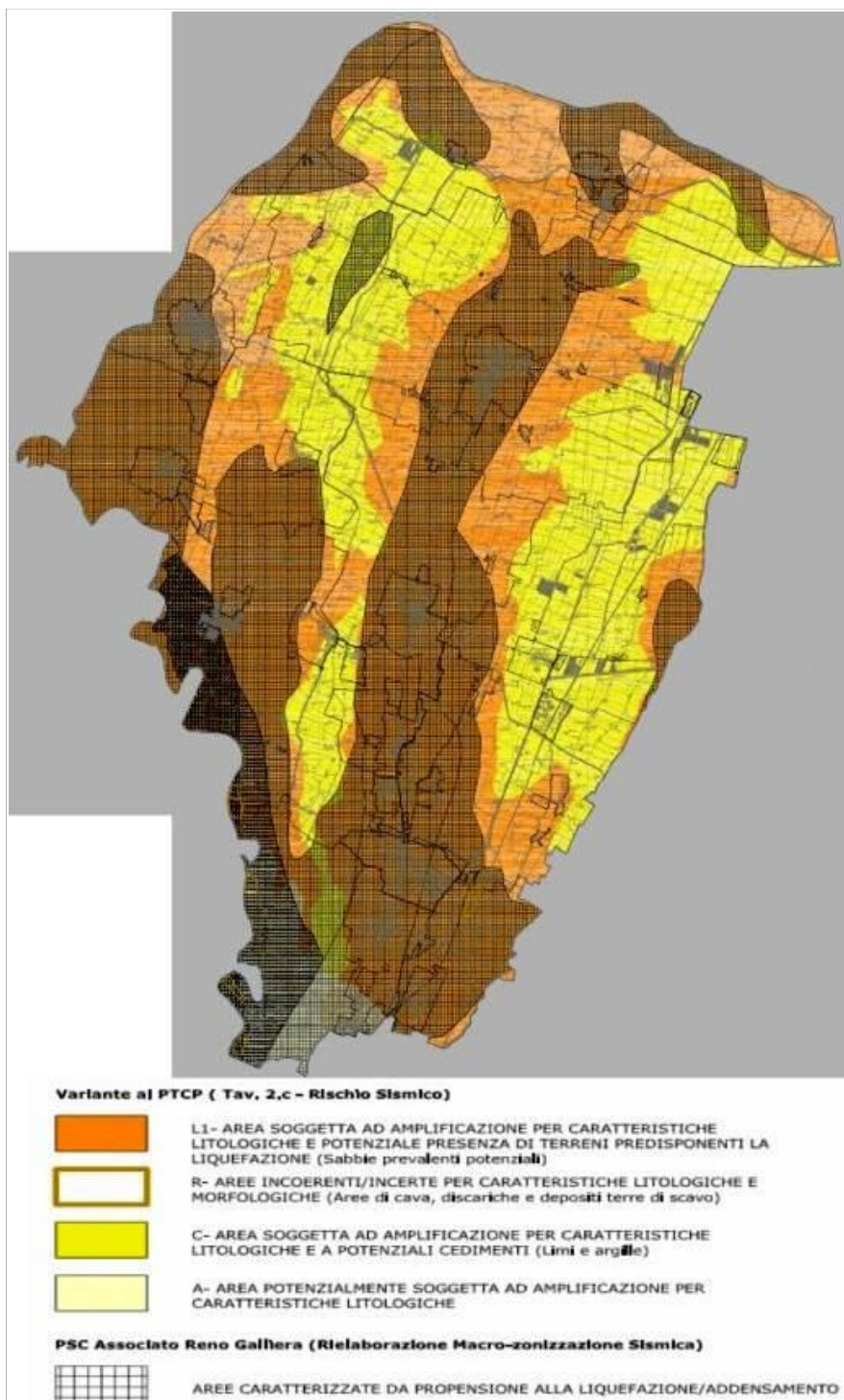
Figura 2.9 – Stralcio della Tav. A del PSC in forma associata dell'Unione Reno-Galliera (scala 1:25.000) – Variante 2013. La cartografia riporta la zonizzazione sismica preliminare del PTCP di Bologna e le zone potenzialmente liquefacibili desunte dal Quadro Conoscitivo del PSC associato
