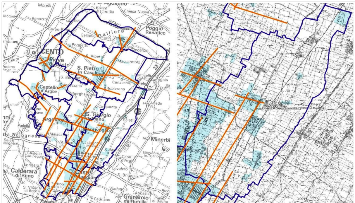
Figura 5.3 – Sezioni litotecniche di riferimento per lo studio di MS (Unione Reno Galliera e dettaglio di Bentivoglio)
