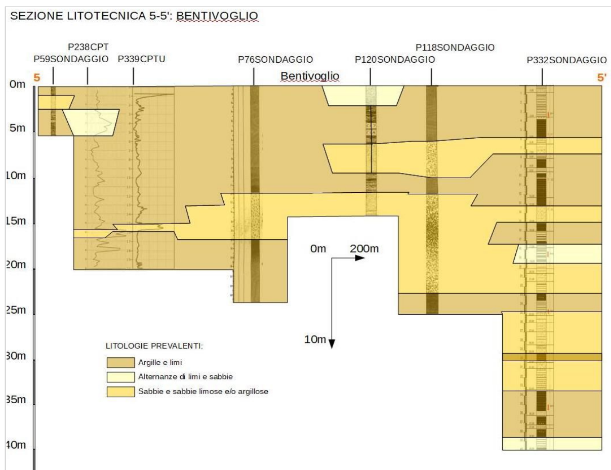
Figura 5.5- Sezione litotecnica 5-5' (Capoluogo) elaborata per questo studio
