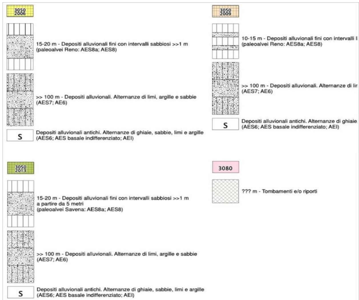
Figura 8.2 – Schemi dei rapporti stratigrafici rappresentativi delle zone di attenzione per instabilità
