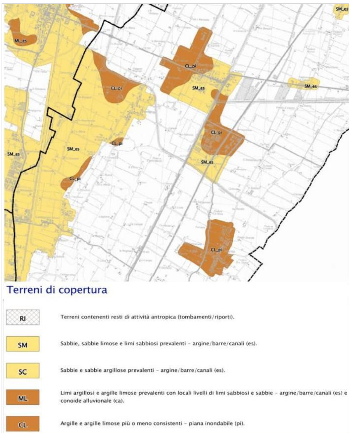
Figura 5.1 – Cartografia geotecnica di sintesi relativa al territorio comunale di Bentivoglio
