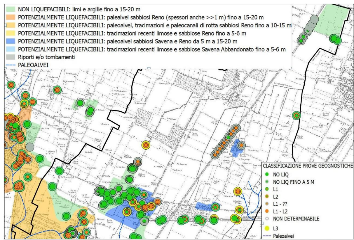
Figura 6.3 - Classificazione dei punti di controllo geognostici finalizzata alla ricostruzione delle zone di potenziale liquefabilità in base alla presenza di strati granulari in falda (territorio NORD)
