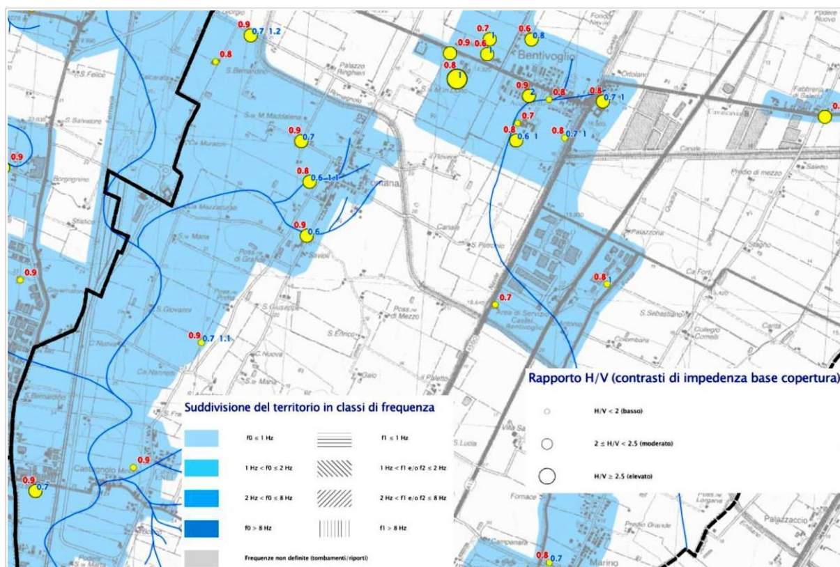
Figura 5.10 – Suddivisione del territorio urbano/urbanizzabile di Bentivoglio in classi di frequenza naturale dei terreni. I colori rappresentano classi differenti. L'ampiezza dei cerchi classifica le massime amplificazioni spettrali ricavate dalle registrazioni HVSR
