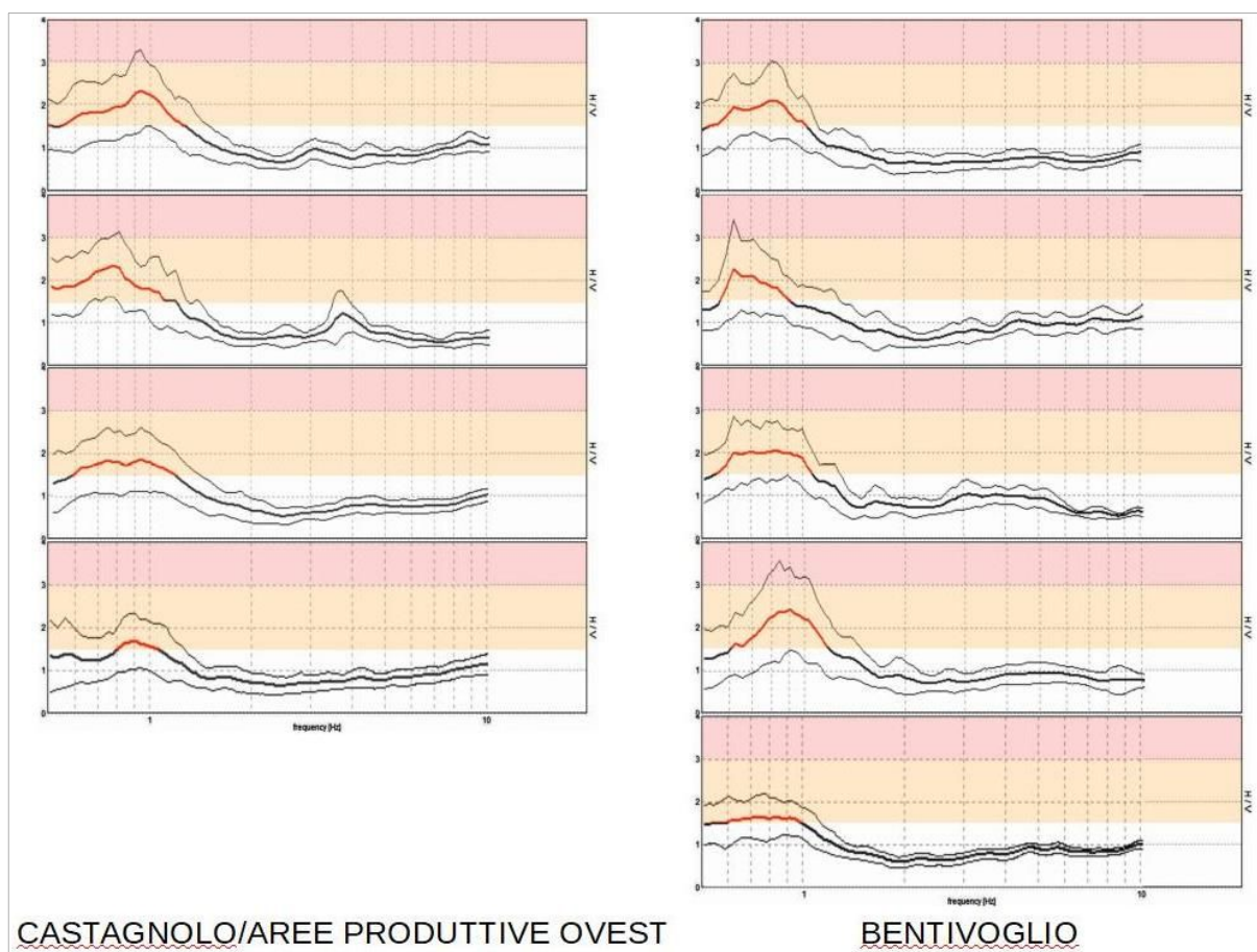
Figura 5.11 - Confronto tra spettri H/V ricavati da registrazioni HVSR nel Comune di Bentivoglio
