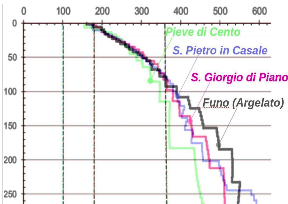
Figura 5.7- Confronto tra alcune sismostratigrafie ESAC elaborate per l'aggiornamento della microzonazione sismica dei Comuni dell'Unione Reno Galliera
