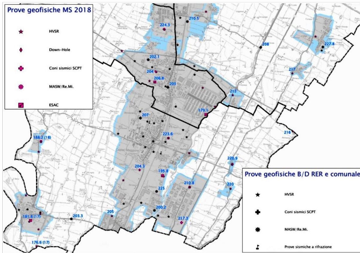
Figura 5.9 - Indagini geofisiche disponibili nel territorio di Castel Maggiore con calcolo della V_{s30} . È indicata anche la tipologia di prova
