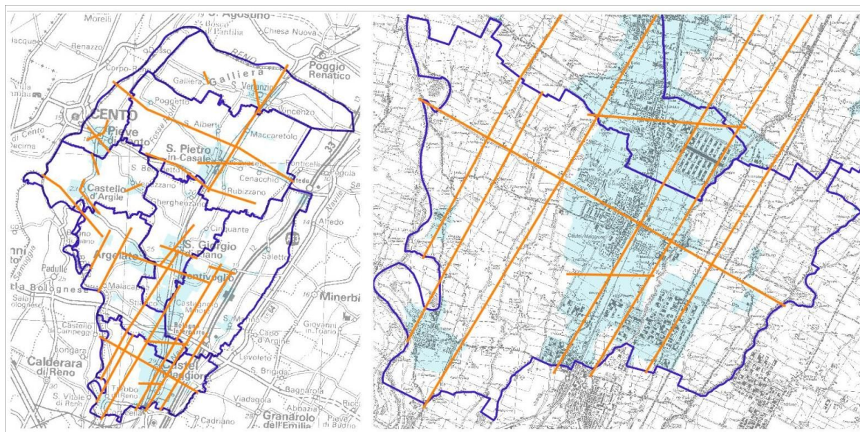
Figura 5.3 – Sezioni litotecniche di riferimento per lo studio di MS (Unione Reno Galliera e dettaglio di Castel Maggiore)
