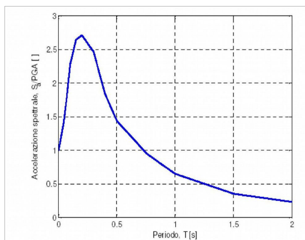
Figura 2.8- Spettro di risposta normalizzato (periodo di ritorno 475 anni; smorzamento 5%) di riferimento per gli studi di MS dell'Emilia-Romagna (DGR 2193/2015)
