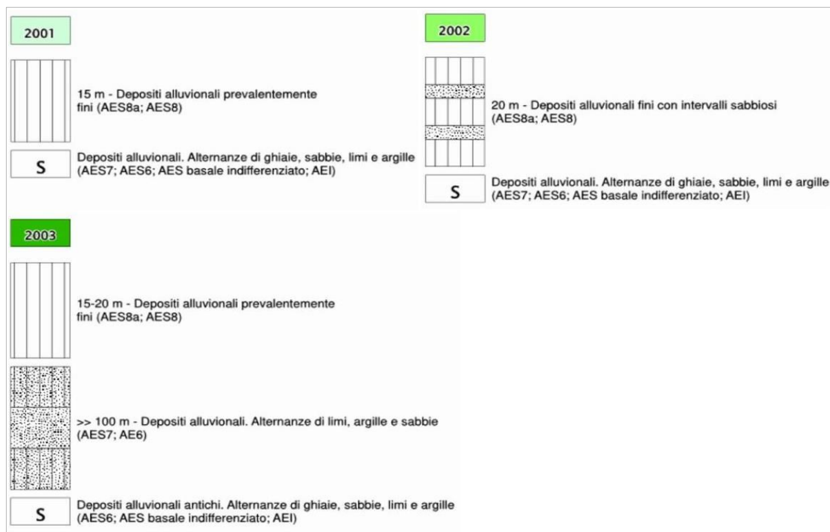
Figura 8.1 - Schemi dei rapporti stratigrafici rappresentativi delle zone stabili
