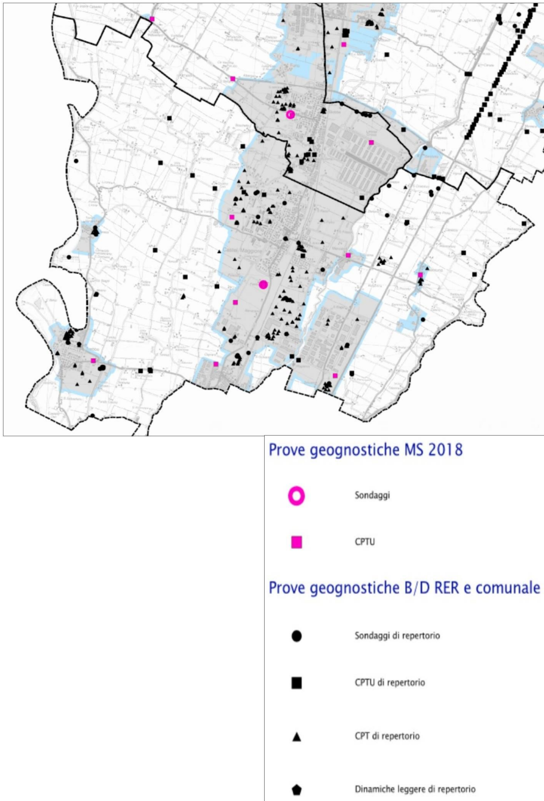
Figura 4.1- Localizzazione delle indagini geognostiche (di repertorio e di nuova esecuzione) disponibili per lo studio di microzonazione sismica
