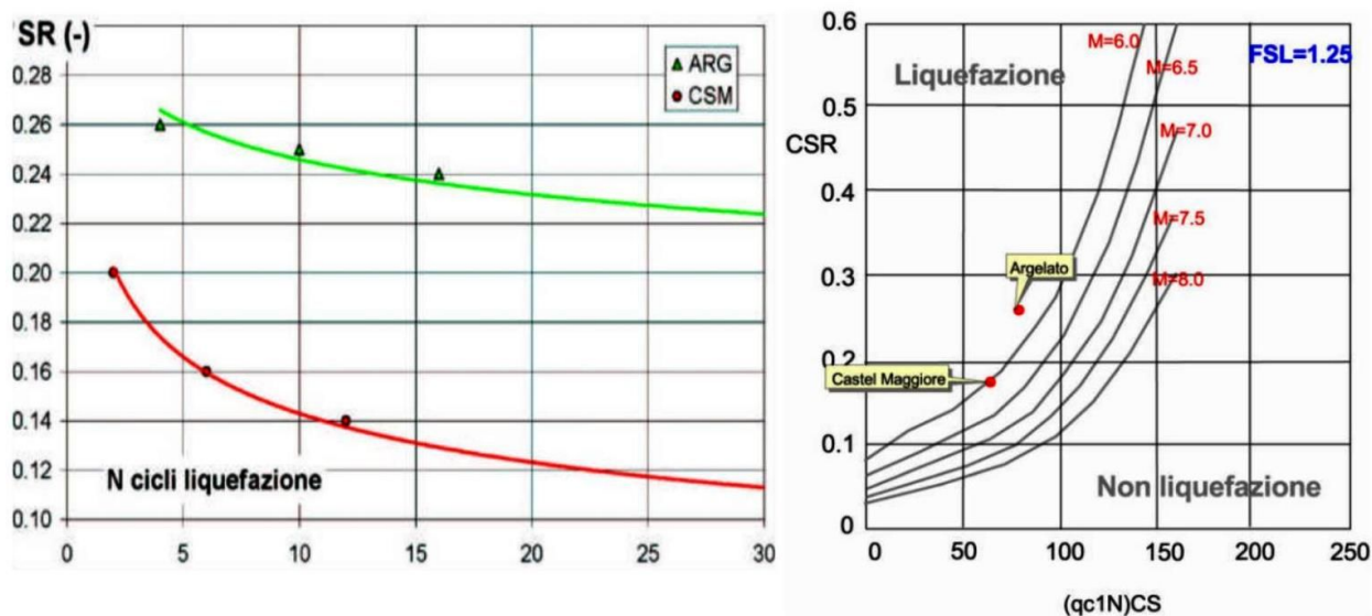
Figura 6.4 - A sx: curve "stress ratio - numero di cicli" ricavate dalle prove triassiali cicliche su campioni prelevati da sondaggi a Castel Maggiore e Funo di Argelato (MS 2008). A dx: correlazione tra CSR e (Qc1N)CS ricavato da prove penetrometriche CPTe/CPTU eseguite in prossimità dei sondaggi
