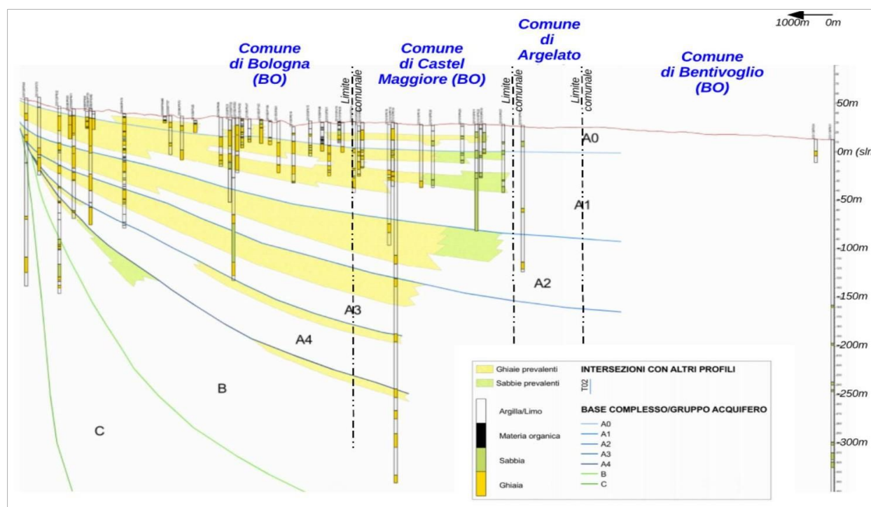
Figura 5.4 – Sezione litotecnica RER (rinominata 3-3' per questo studio)
