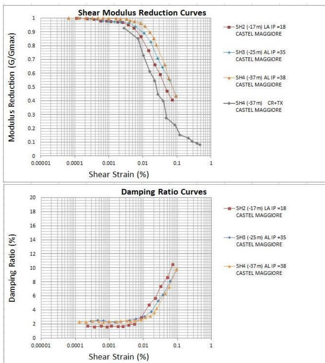
Figura 5.2 - Curve di decadimento dei sedimenti fini di Castel Maggiore (sondaggio eseguito nel Capoluogo)
