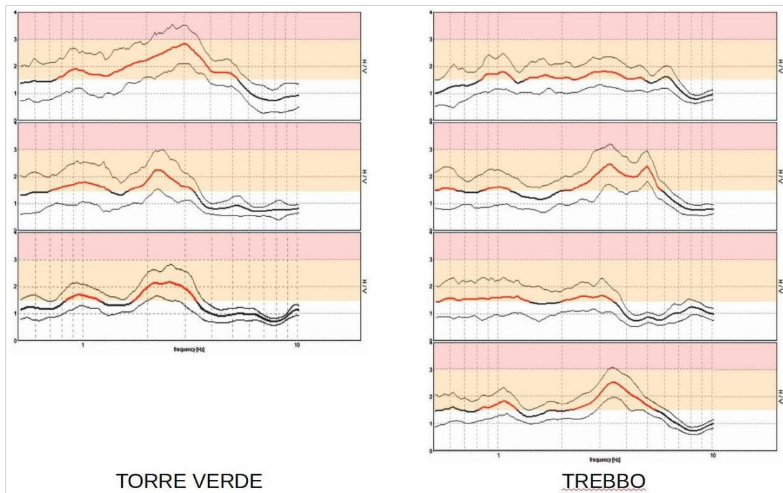
Figura 5.12 - Confronto tra spettri H/V ricavati da registrazioni HVSR eseguite a Castel Maggiore (Trebbio; Torre Verde)
