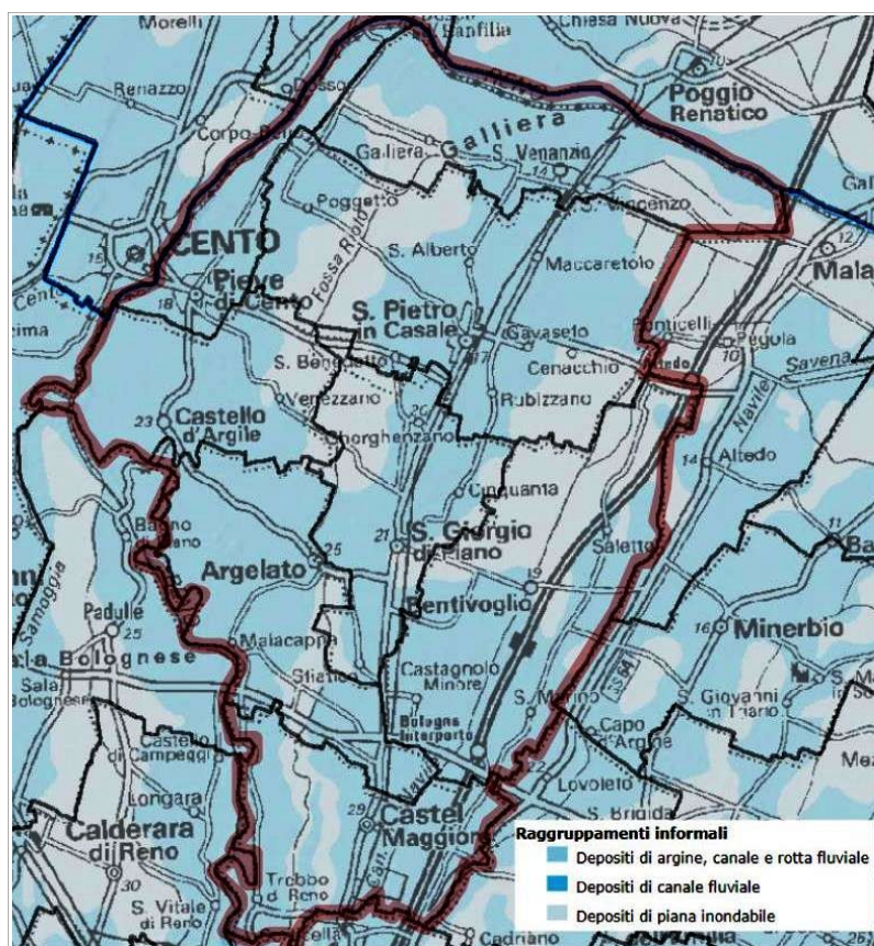
Figura 3.6 - Geologia di sintesi dei depositi affioranti classificati in relazione alla facies deposizionale (fonte: cartografia geologica interattiva pubblicata nel sito internet del SGSS regionale)
