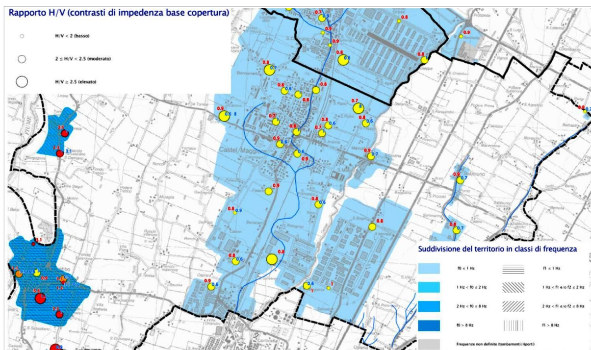
Figura 5.10 – Suddivisione del territorio urbano/urbanizzabile di Castel Maggiore in classi di frequenza naturale dei terreni. I colori rappresentano classi differenti. L'ampiezza dei cerchi classifica le massime amplificazioni spettrali ricavate dalle registrazioni HVSR
