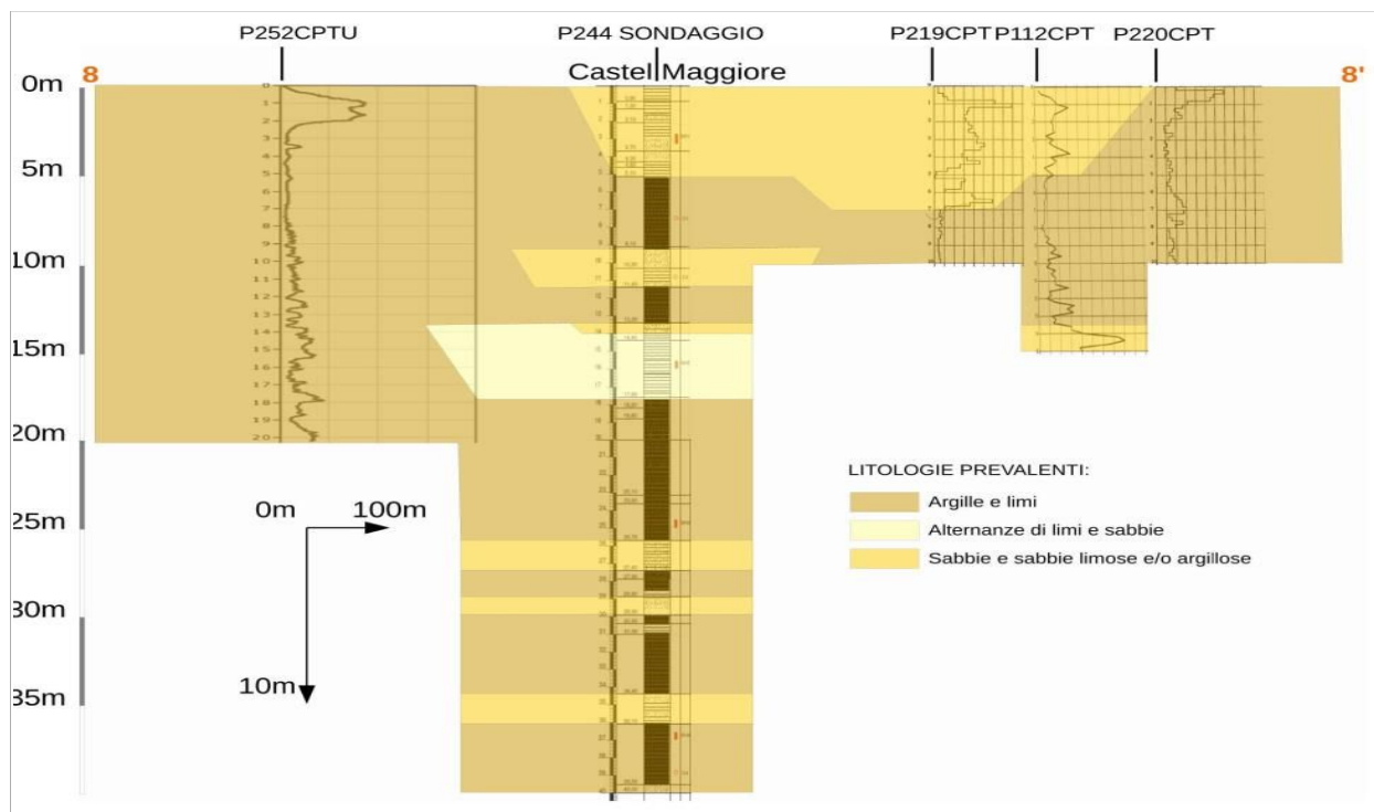
Figura 5.5- Sezione litotecnica 8-8' (Capoluogo) elaborata per questo studio
