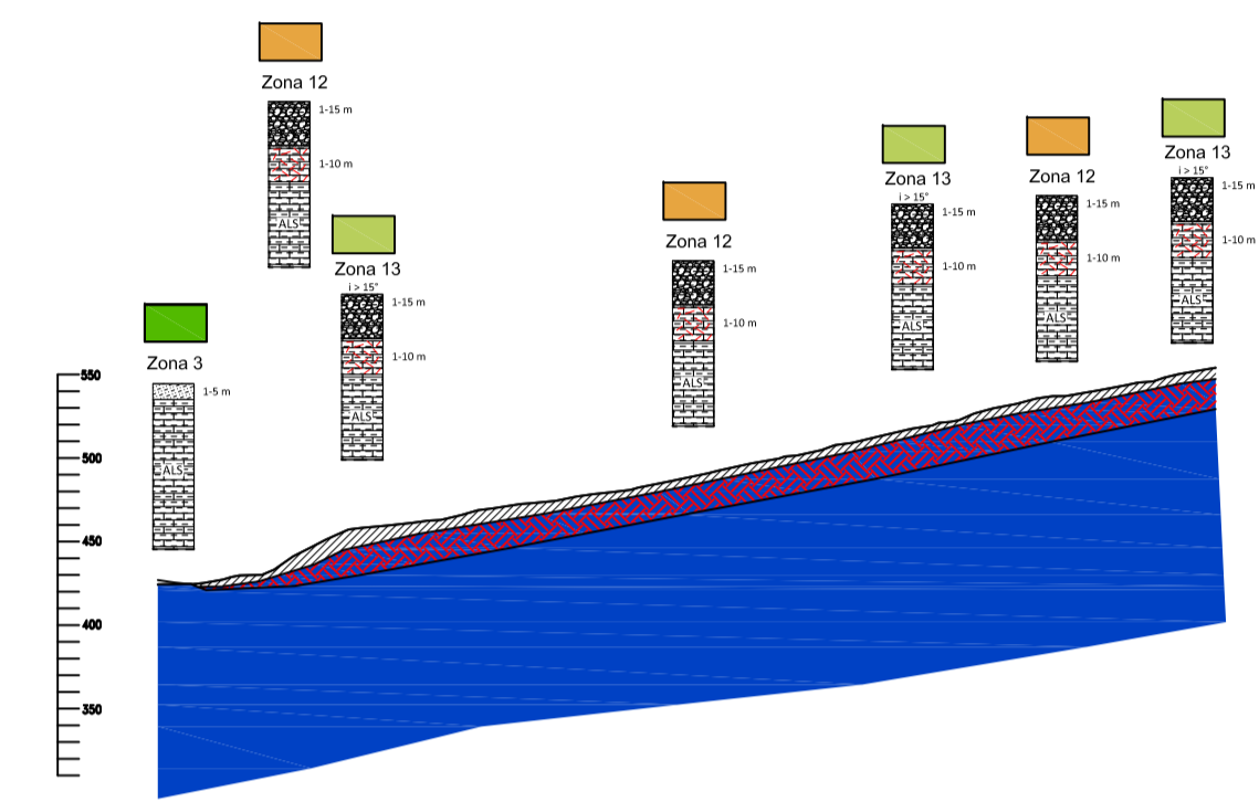
SEZIONE 7
