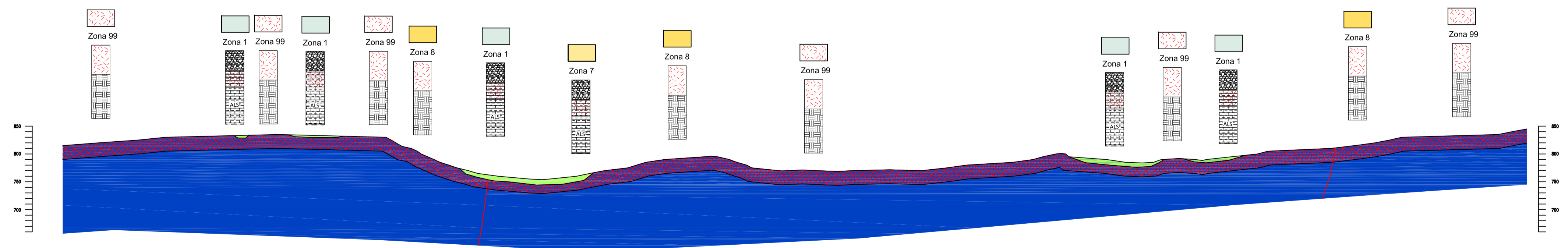
SEZIONE 1a
