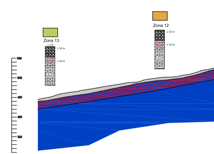
SEZIONE 6
