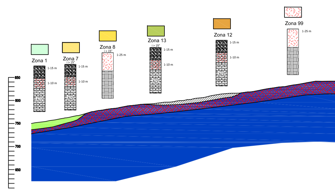
SEZIONE 1
