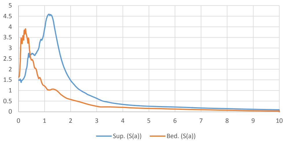
Spettro in accelerazione Sez11_nodo234
