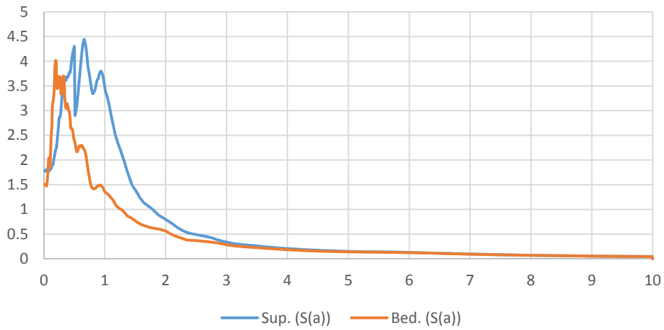
Spettro in accelerazione Sez8_nodo564
