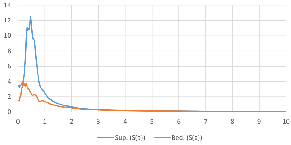
Spettro in accelerazione Sez4_nodo443
