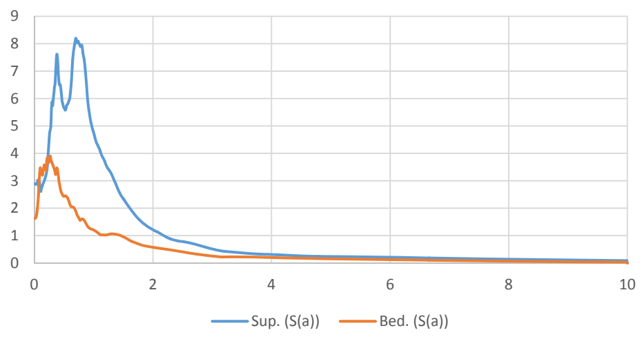
Spettro in accelerazione Sez8_nodo516
