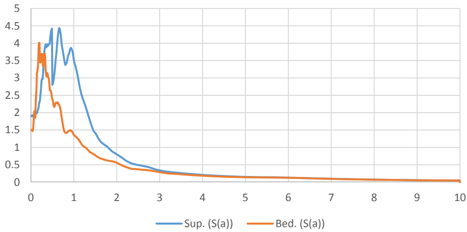
Spettro in accelerazione Sez8_nodo581
