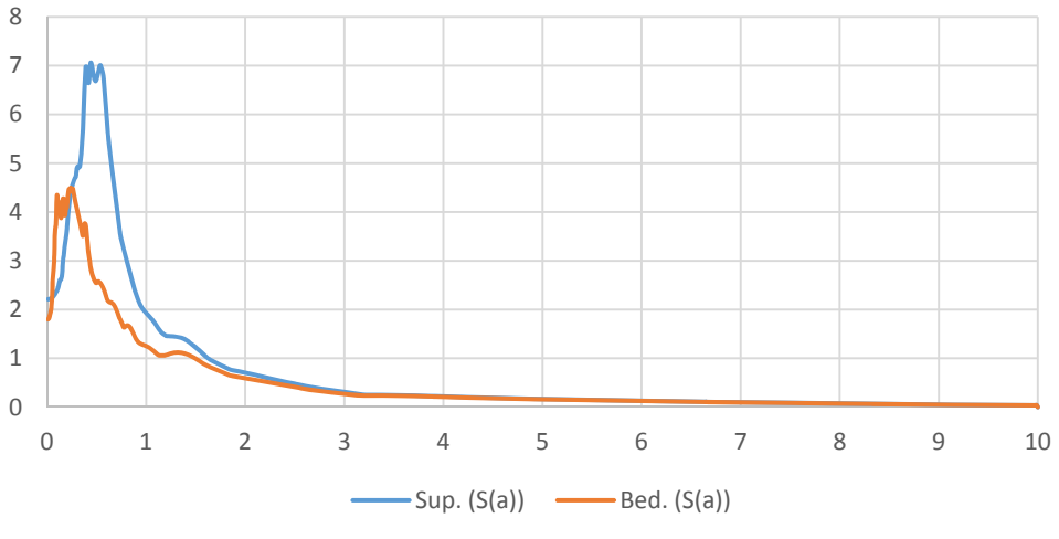
Spettro in accelerazione Sez1_nodo661
