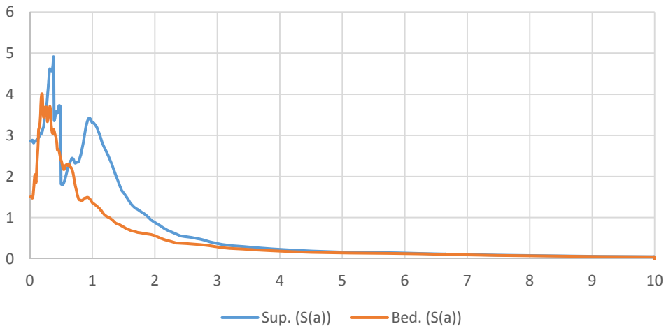
Spettro in accelerazione Sez9_nodo173
