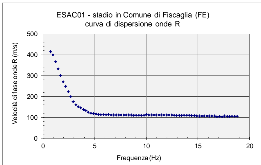
Figura 3. Curva di dispersione delle onde Rayleigh del profilo sismico ESAC01.
