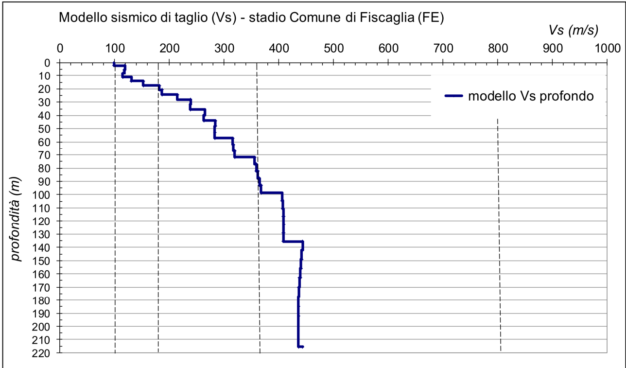
Figura 5. Il profilo verticale VS ottenuto per l’area indagata dal profilo sismico. In base al modello sismico è stata determinata la VS30 che risulta pari a 146 \text{ m/s} \pm 4 \text{ m/s} (RMS=1.5%).
