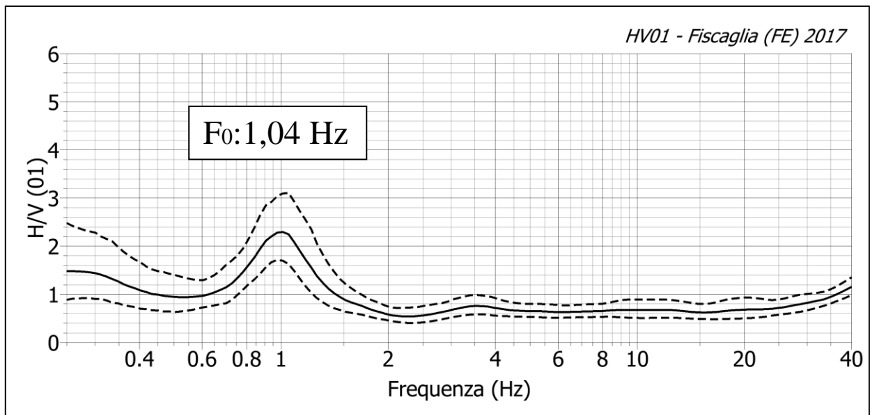
Figura 7. Spettro medio dei rapporti spettrali (H/V) effettuate in campo libero della prova n. 01 acquisita nella vicinanza dello stadio di Fiscaglia (FE). Le frecce indicano le frequenze di risonanza tipiche dei terreni investigati. F0: frequenza di risonanza dei terreni.
