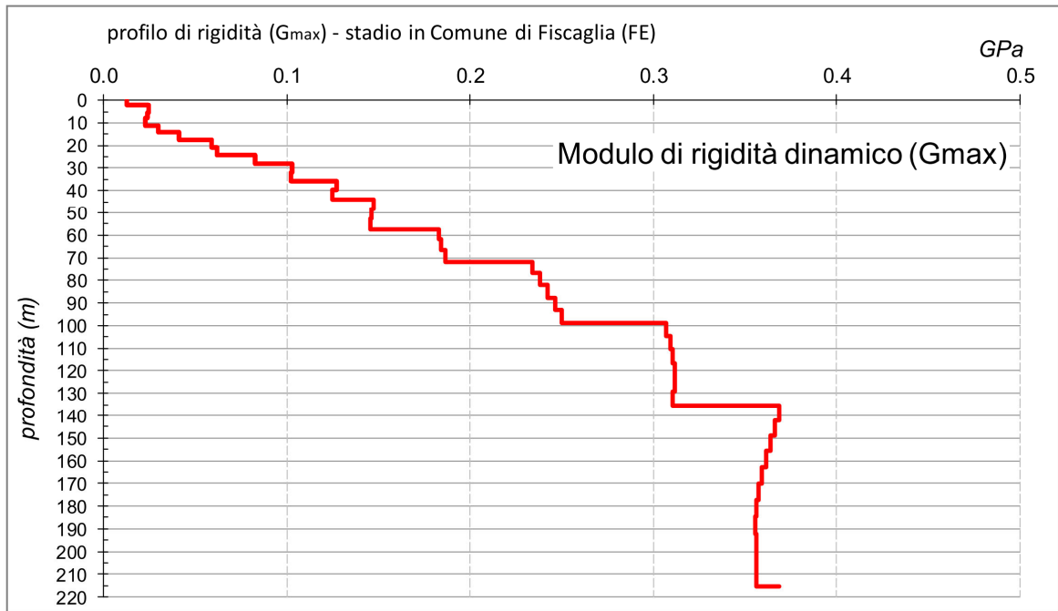
Figura 6. Il profilo verticale G_{max} ( \mu : modulo di rigidità dinamico) dell'area indagata dal profilo sismico, ottenuto dal profilo di velocità ( V_s ) mediante l'equazione \mu = \rho \cdot V_s^2 .
