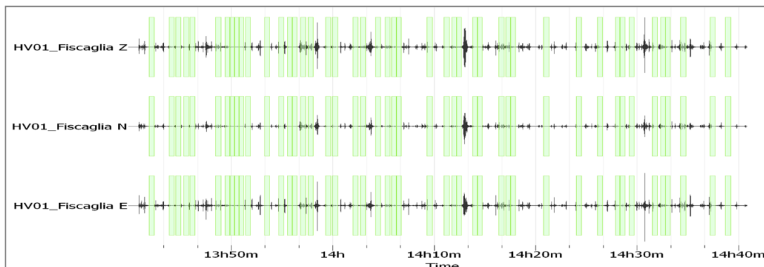
Figura 4. Sismogramma del data set di rumore sismico acquisito in campo libero a Fiscaglia (HV01). Z: componente verticale, N: componente orizzontale in direzione N-S e E: componente orizzontale in direzione E-W.
