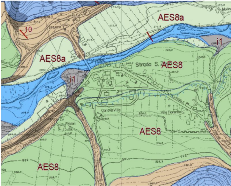
Carta Geologica Regionale –località Strada San Zeno
