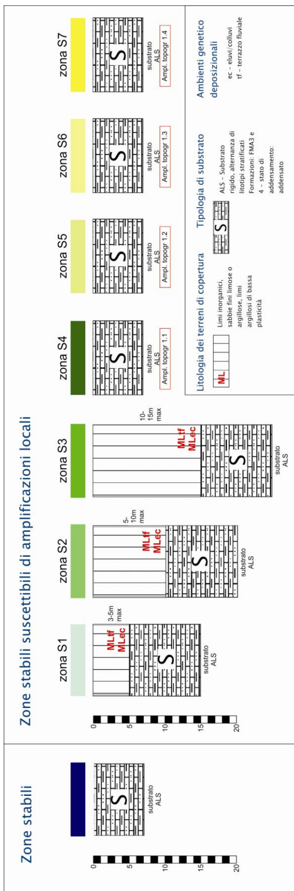
Fig. 5 - Microzone omogenee in prospettiva sismica (MOPS)
