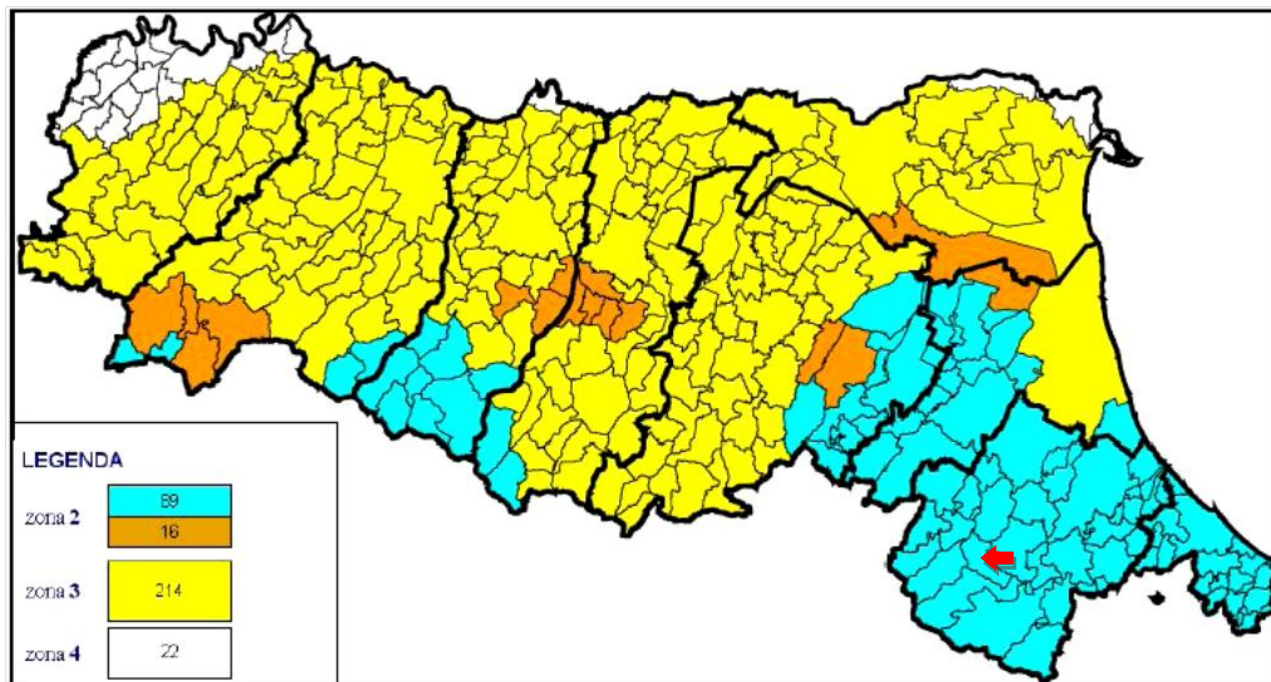
FIG. 2- CLASSIFICAZIONE SISMICA DEI COMUNI DELLA REGIONE EMILIA-ROMAGNA – . (Comune di Galeata ←)
