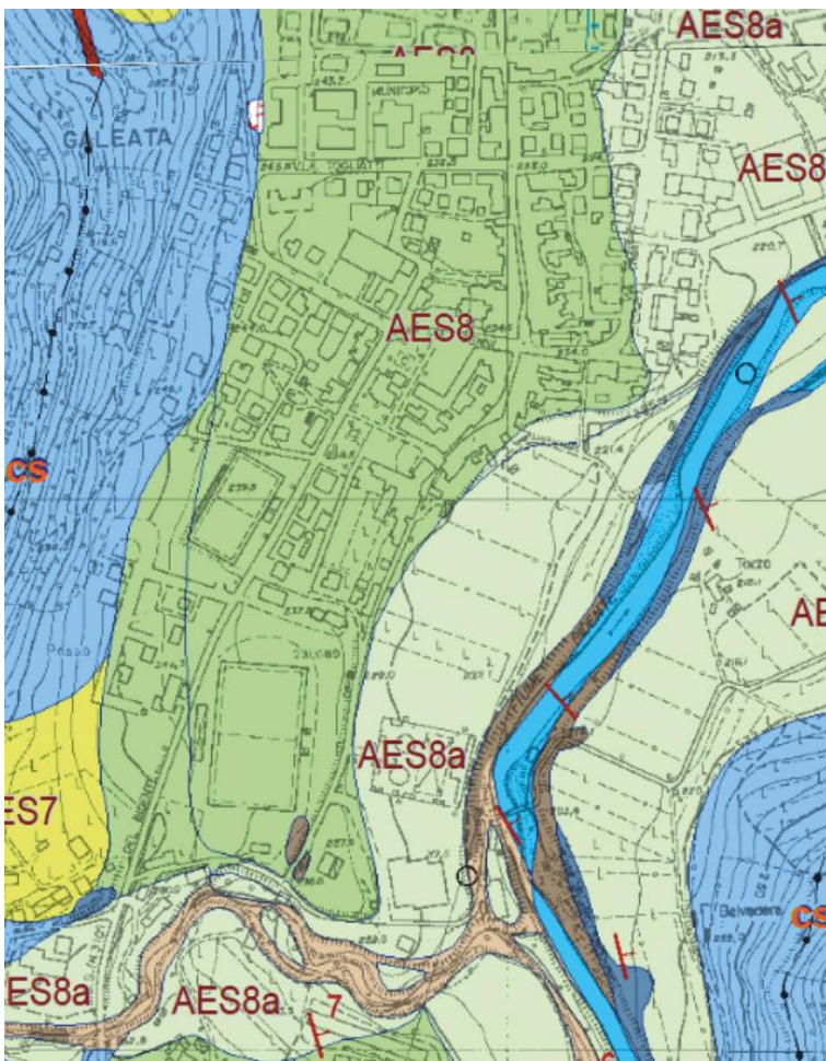
Carta Geologica Regionale –Galeata capoluogo
