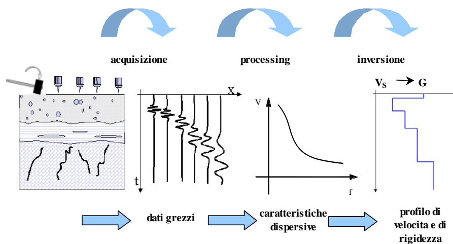
Fig. 2 Fasi del metodo delle onde superficiali (SWM)
