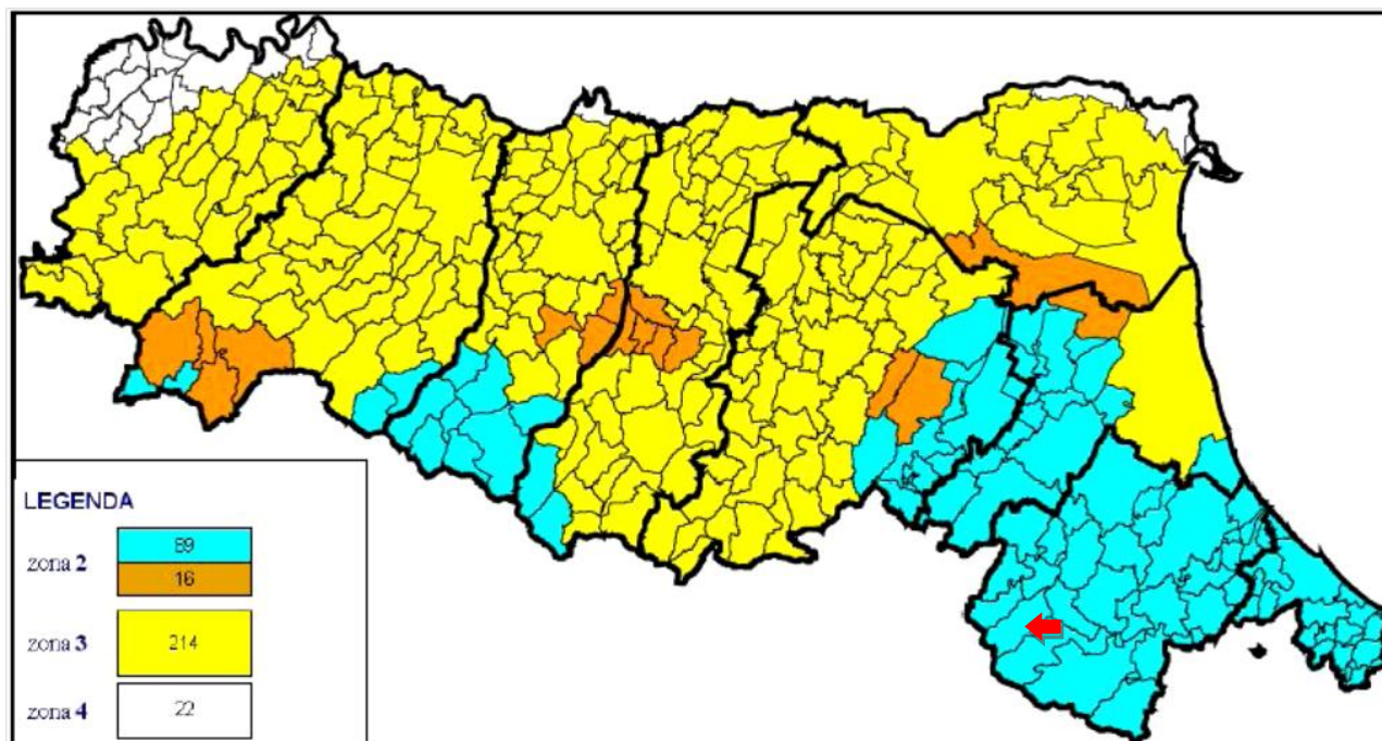
FIG. 2- CLASSIFICAZIONE SISMICA DEI COMUNI DELLA REGIONE EMILIA-ROMAGNA – . (Comune di Premilcuore ←)
