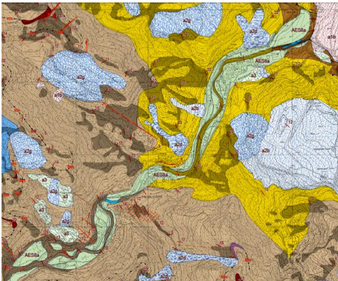
Carta Geologica Regionale – Premilcuore capoluogo
