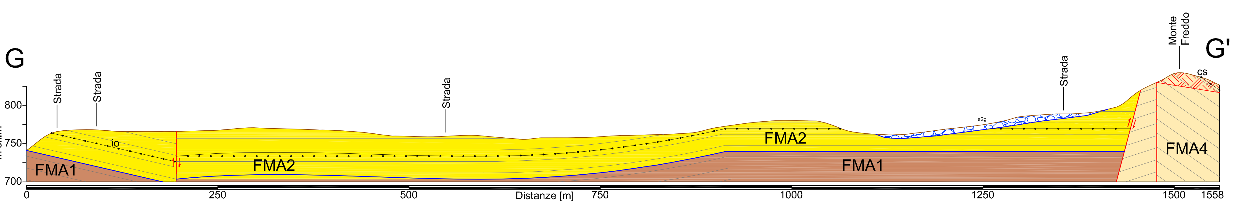
Sezioni geologiche in scala 1:3.000
