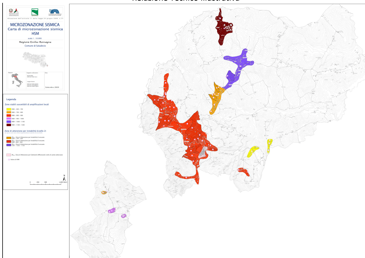
Figura 7.8– Miniatura della carta di scuotimento assoluto H_{SM} , Comune di Saludecio.
