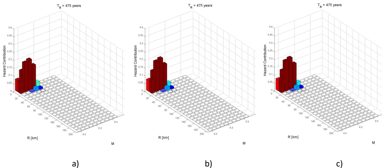
Figura 3.6–Diagramma di disaggregazione riferito all’area di Montescudo (a), Montecolombo (b), Saludecio (c).
