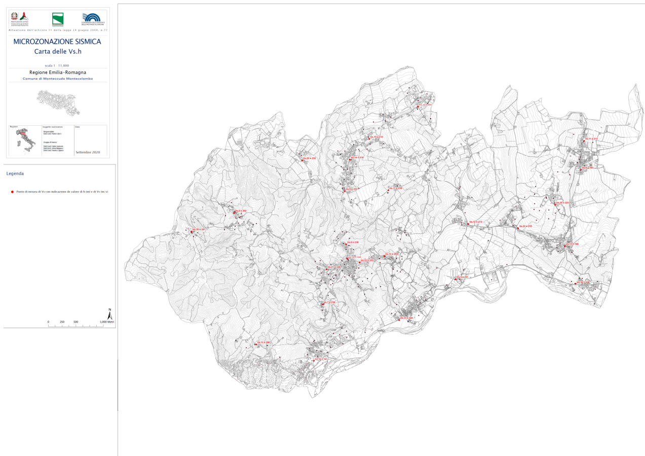
Figura 7.1 – Miniatura della carta delle velocità delle onde di taglio V_sH , Comune di Montescudo-Montecolombo
