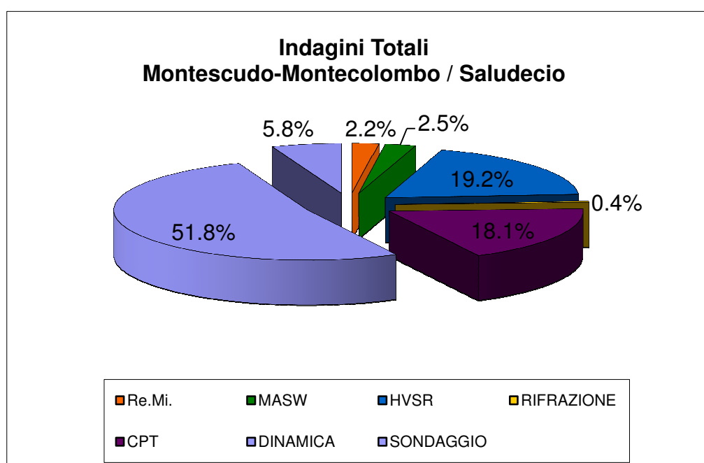
Figura 5.1 – Totale Indagini distribuite sul territorio dell'Unione Comuni della Valconca utilizzate per la MS nei comuni di Montescudo-Montecolombo e Saludecio.
