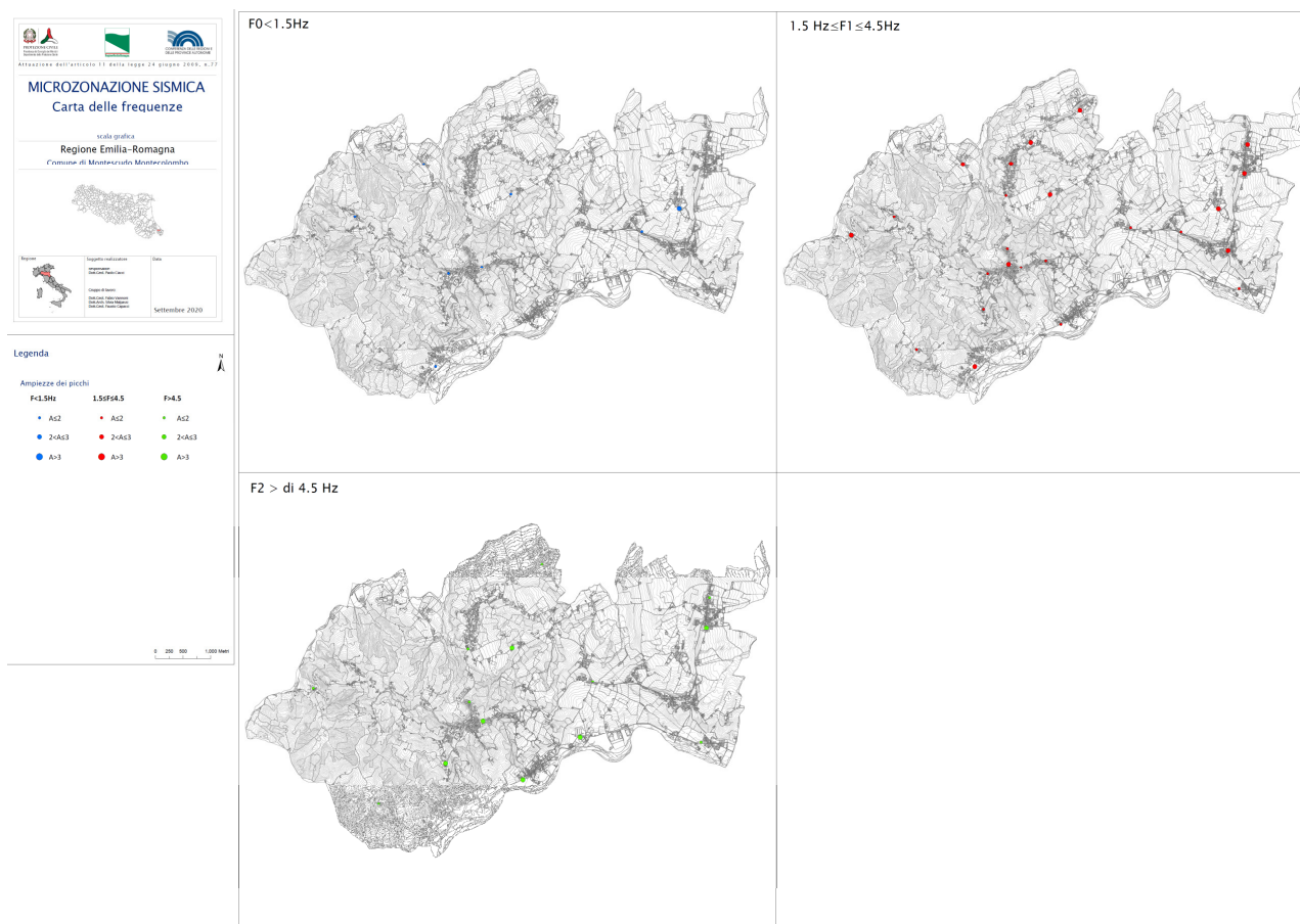
Figura 6.4 – Miniatura della Mappa delle Frequenze Naturali dei Terreni di Montescudo-Montecolombo.
