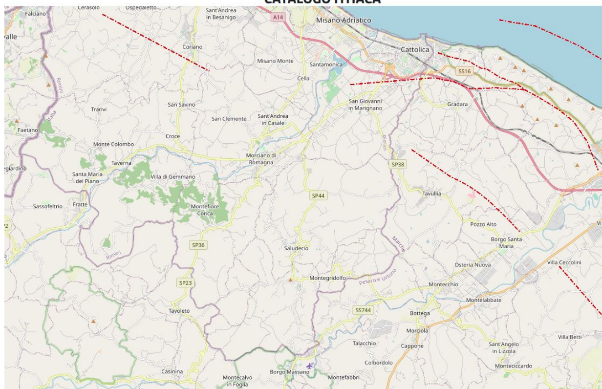
Figura 3.8 – Dettaglio catalogo ITHACA delle faglie attive e capaci.
