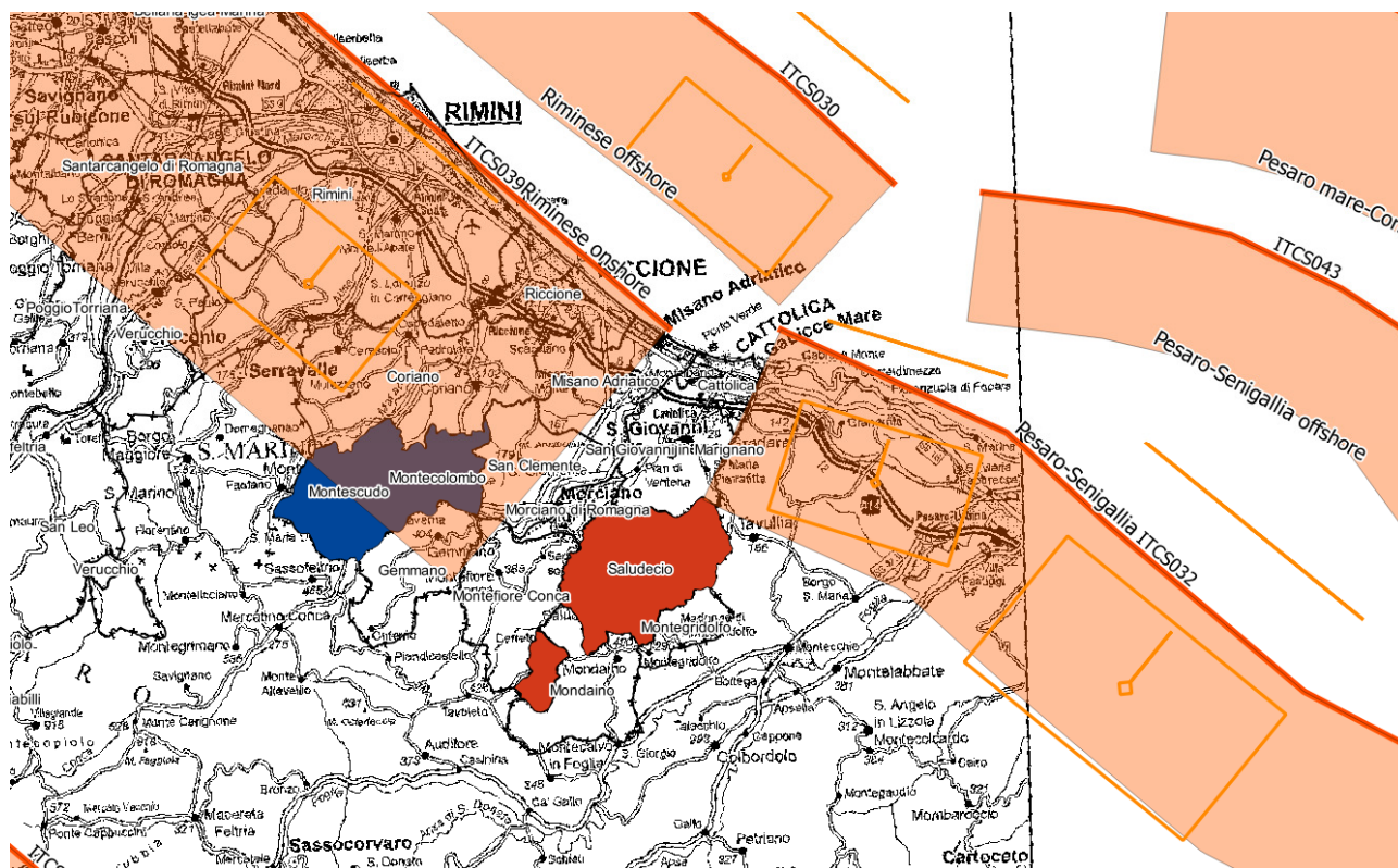
Figura – 3.4: Sorgenti sismogenetiche (Id-Nome-Max Magnitudo) individuate dal catalogo DISS (Database of Individual Seismogenic Sources) dell’Istituto Nazionale di Geofisica e Vulcanologia.
