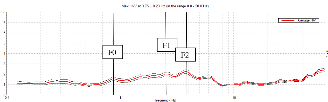
Figura 6.2-Curva dei rapporti spettrali relativa alla registrazione H01 di Saludecio.
