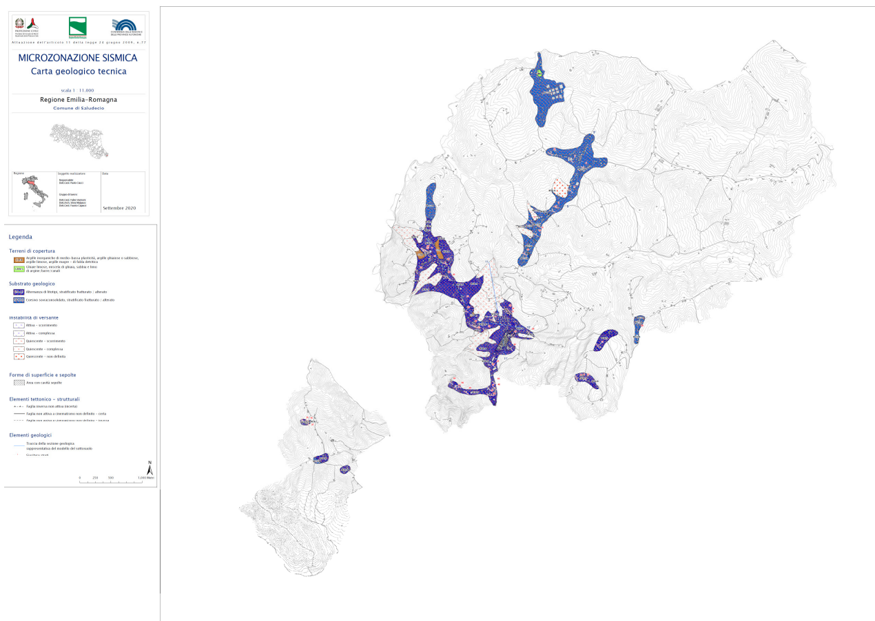
Figura 6.1 – Miniatura della Carta Geologico-Tecnica dell'unione di Comuni della Valconca; Saludecio.
