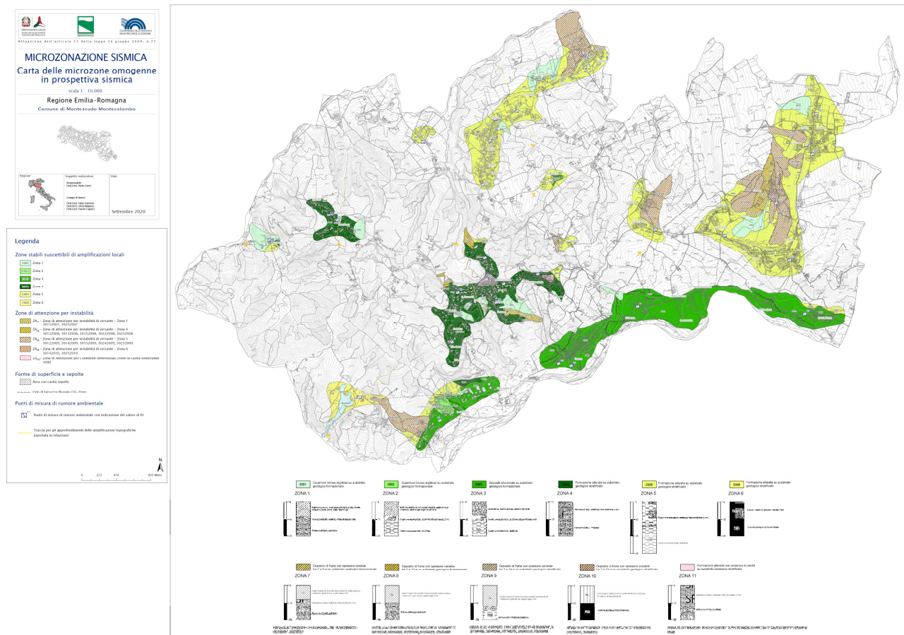
Figura 6.5-Miniatura della Carta delle MOPS riferita al Comune di Montescudo-Montecolombo (RN).
